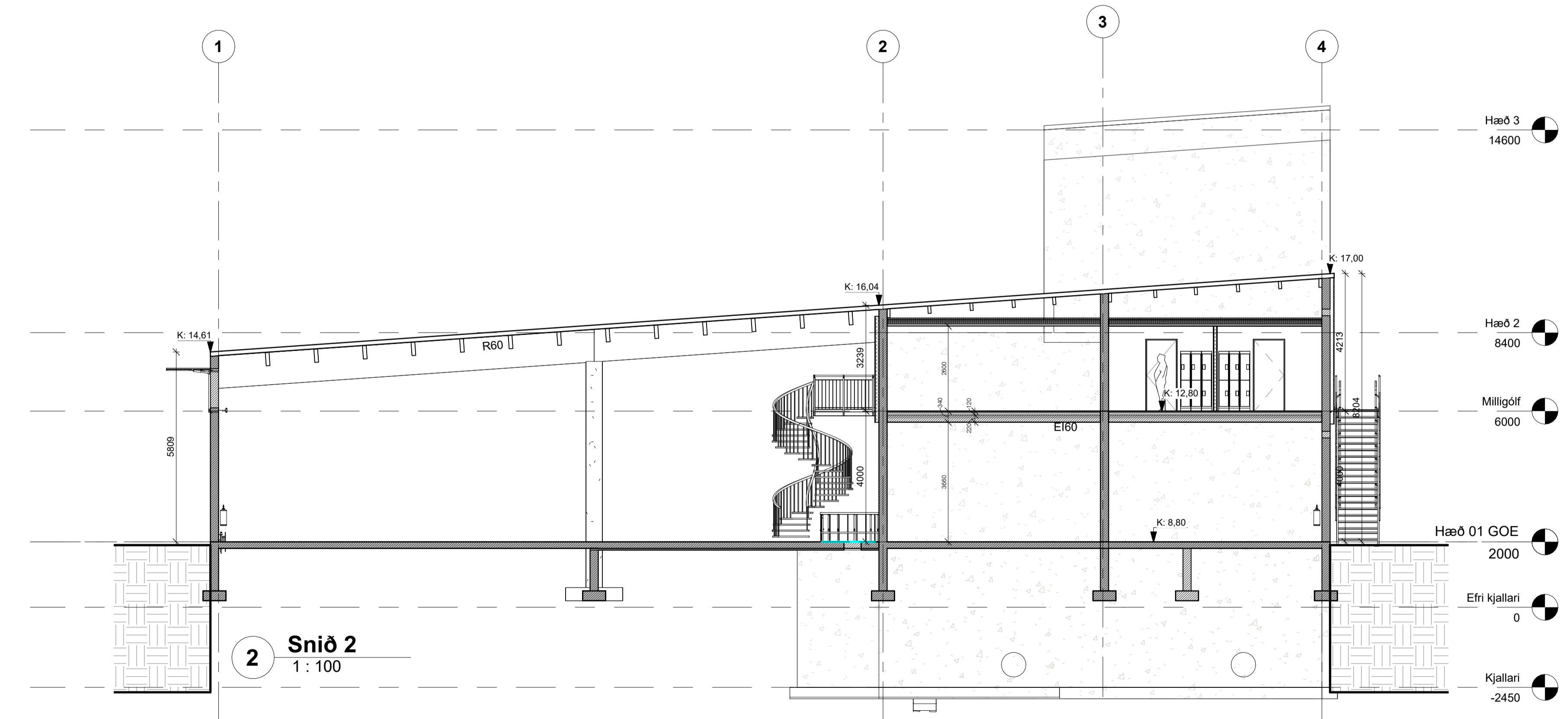
1 Snið 1 1 : 100
