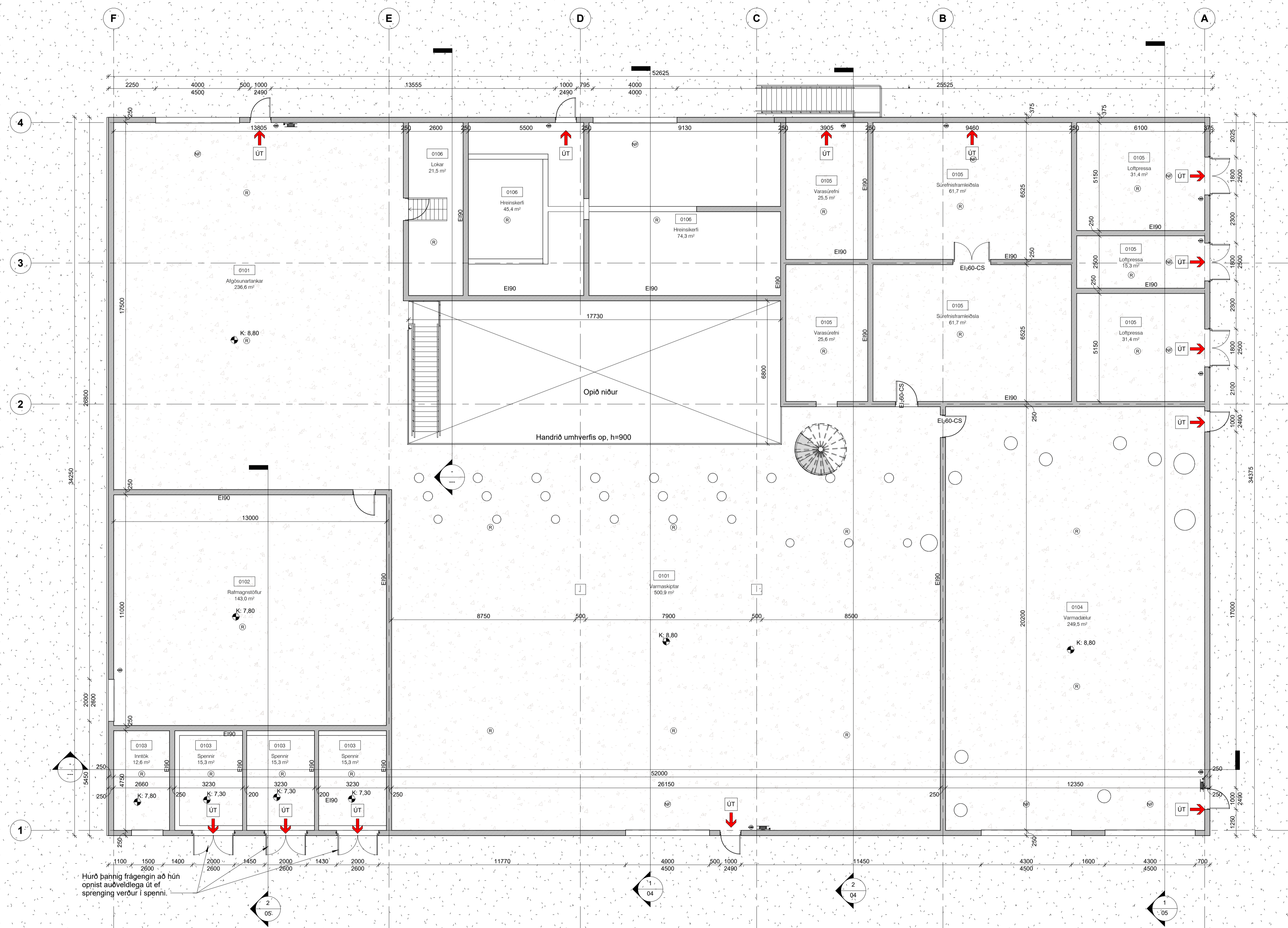
1 Hæð 1 1 : 100
