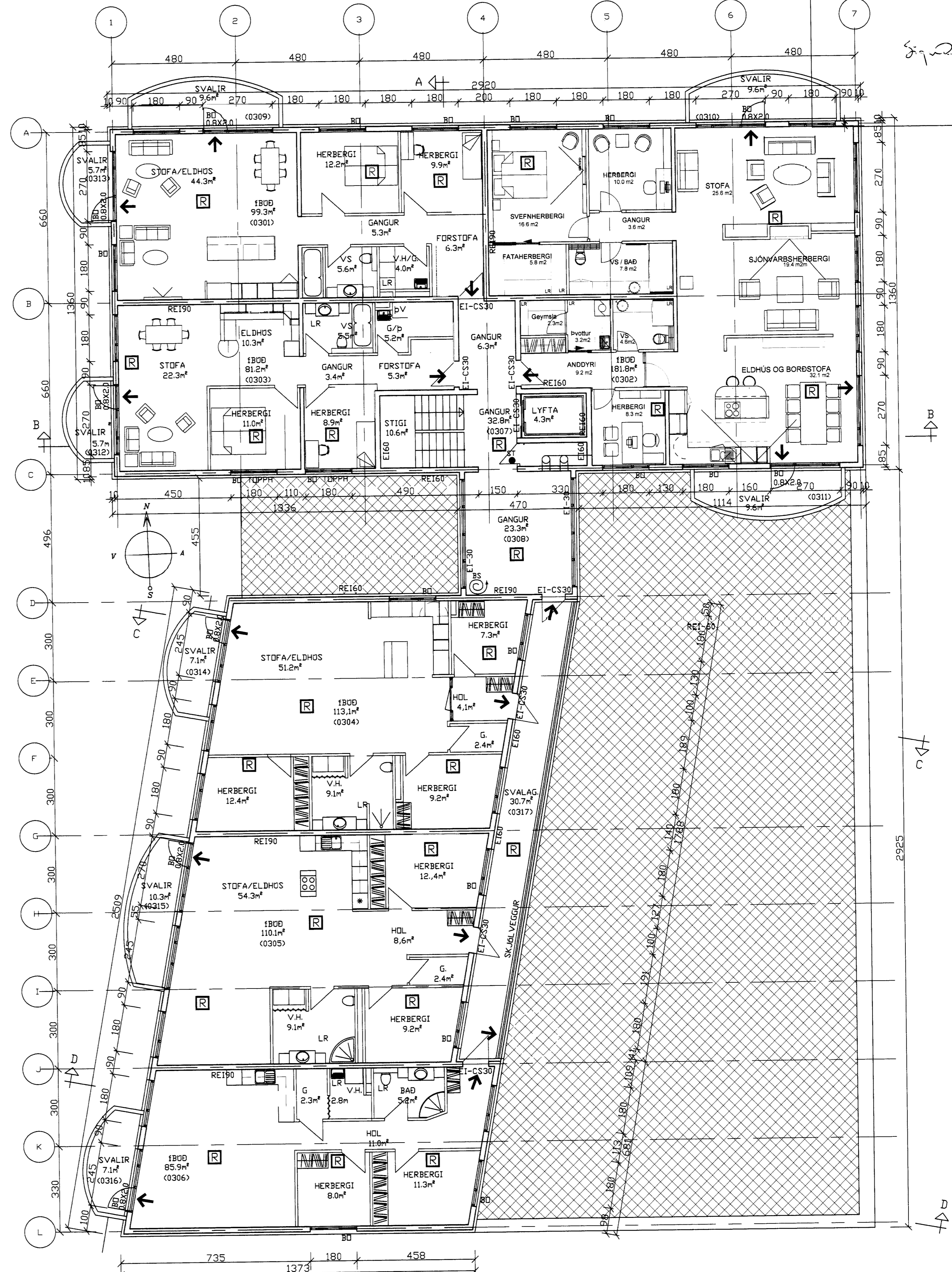
GRUNNMYND 3. HÆÐ
