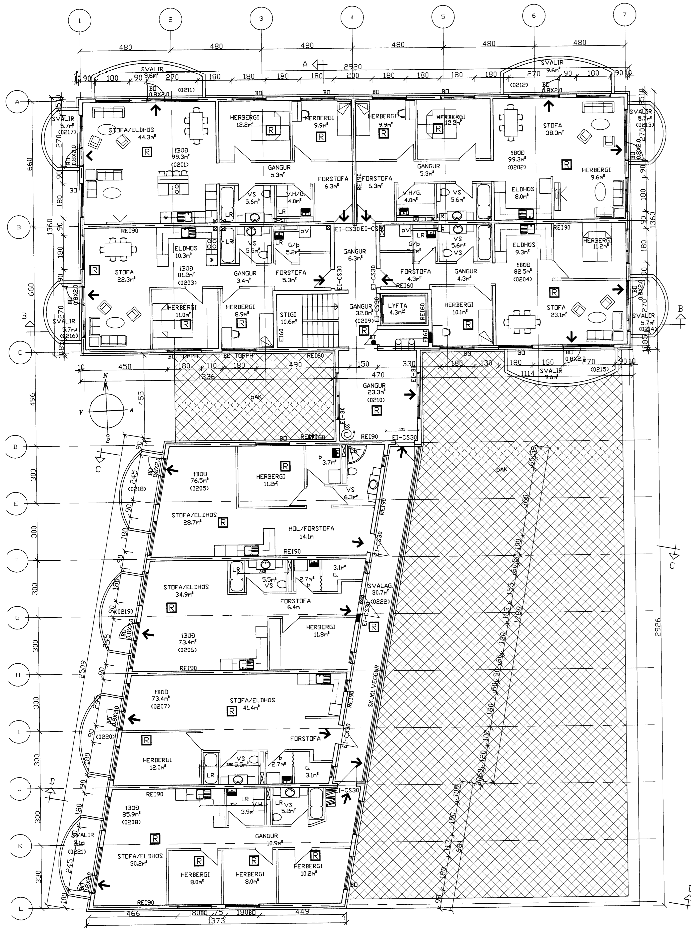
GRUNNMYND 2. HÆÐ
