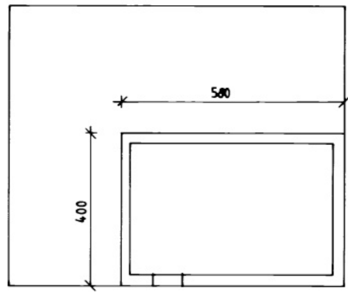
D - D
