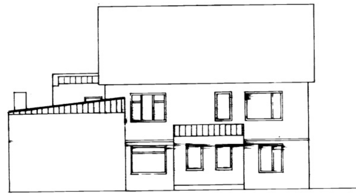
SUÐUR
