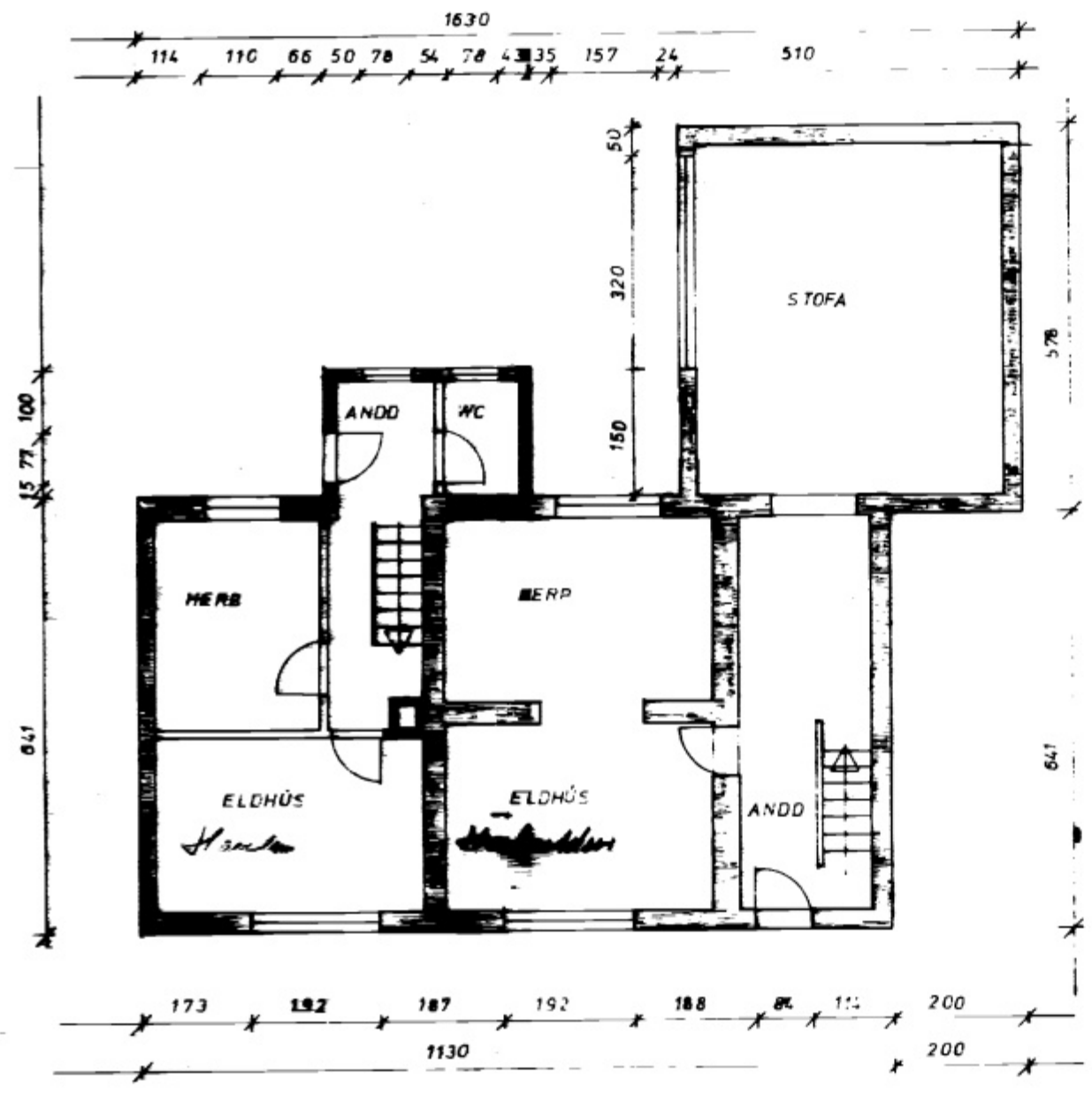
GRUNNMYND 1:100 1 HÆÐ
