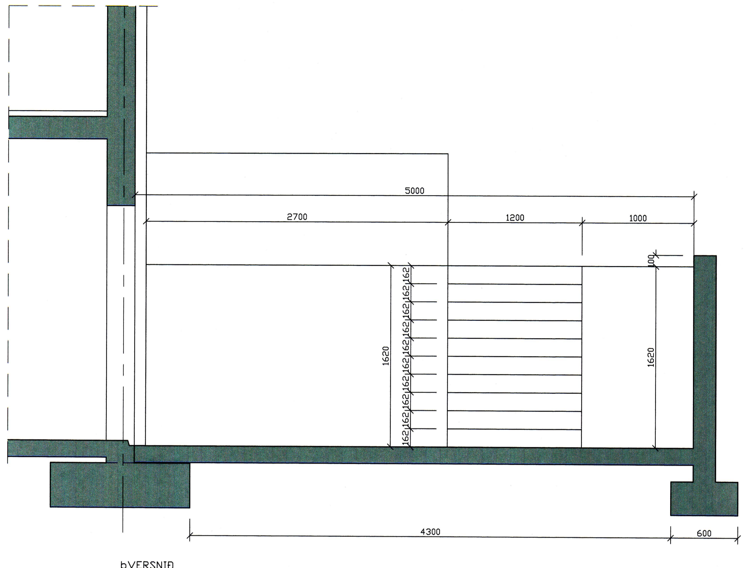
ÞVERSNIÐ
