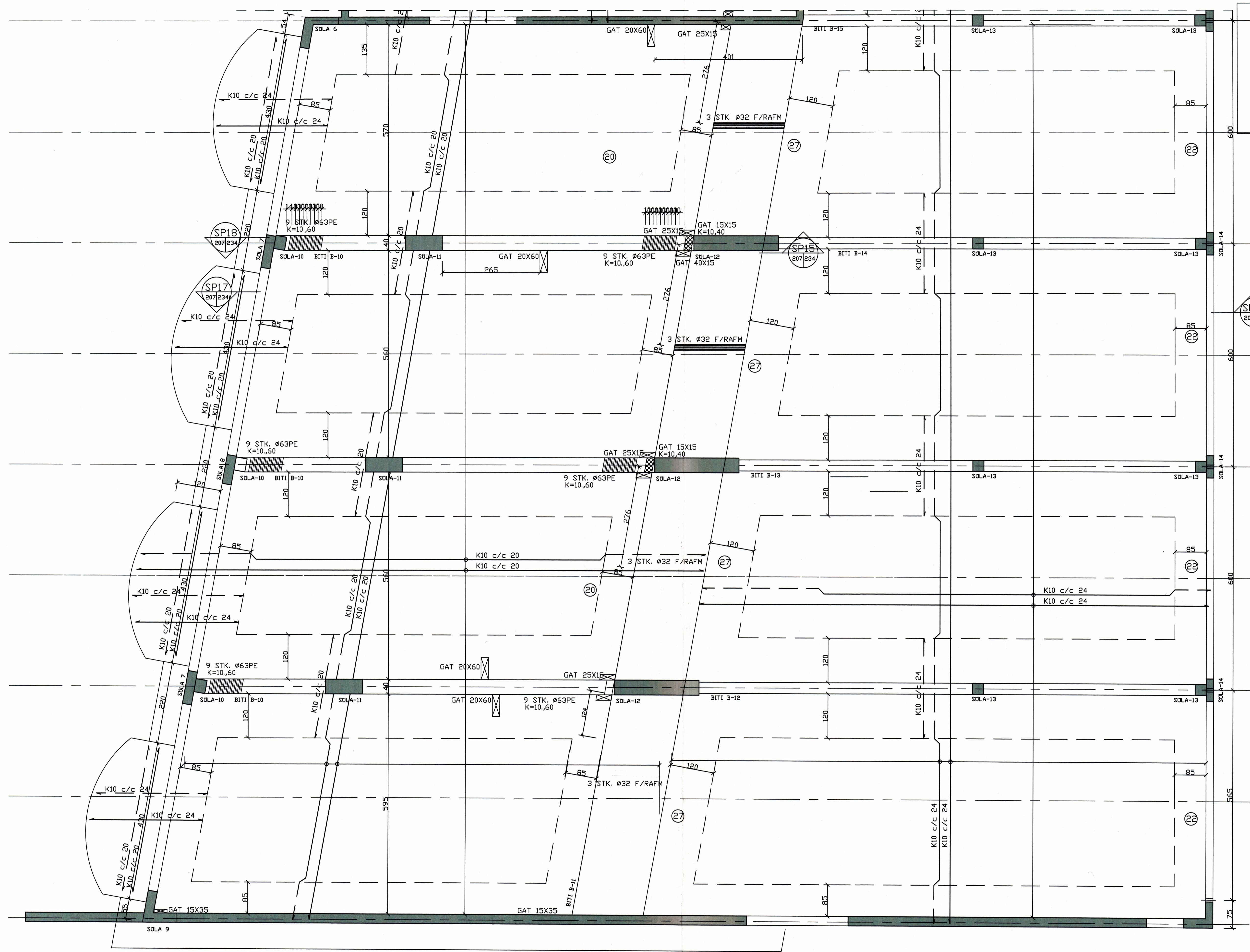
GRUNNMYND PLATA YFIR 1. HÆÐ SUÐURENDI
