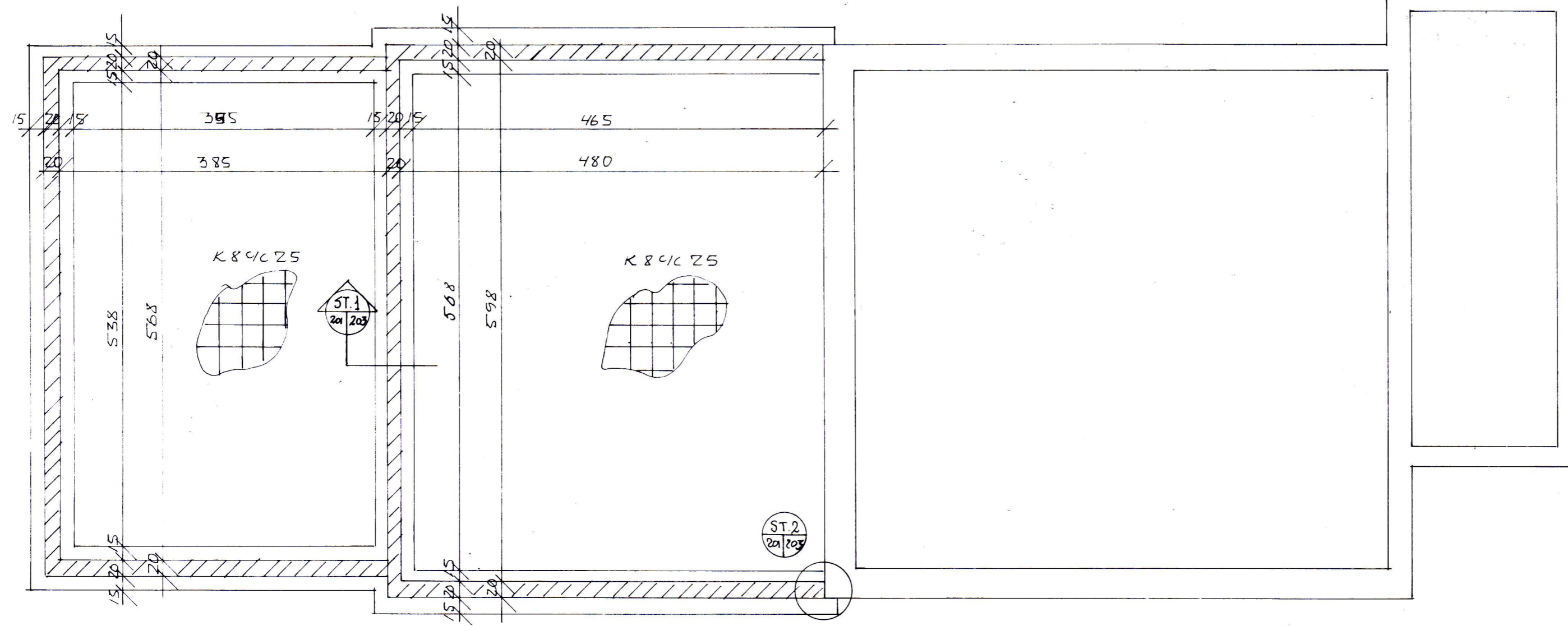
GRUNNMYND SÖKKLAR M = 1:50
