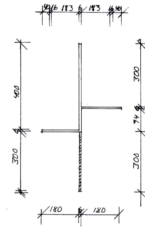
STÁLFASTING FYRIR LIMTRÉ M=1:10
