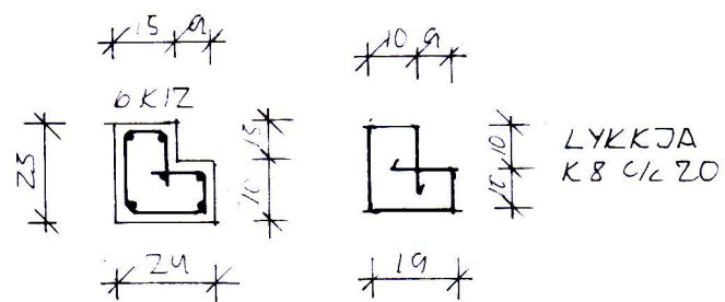
SÚLA S-2 M=1:20
