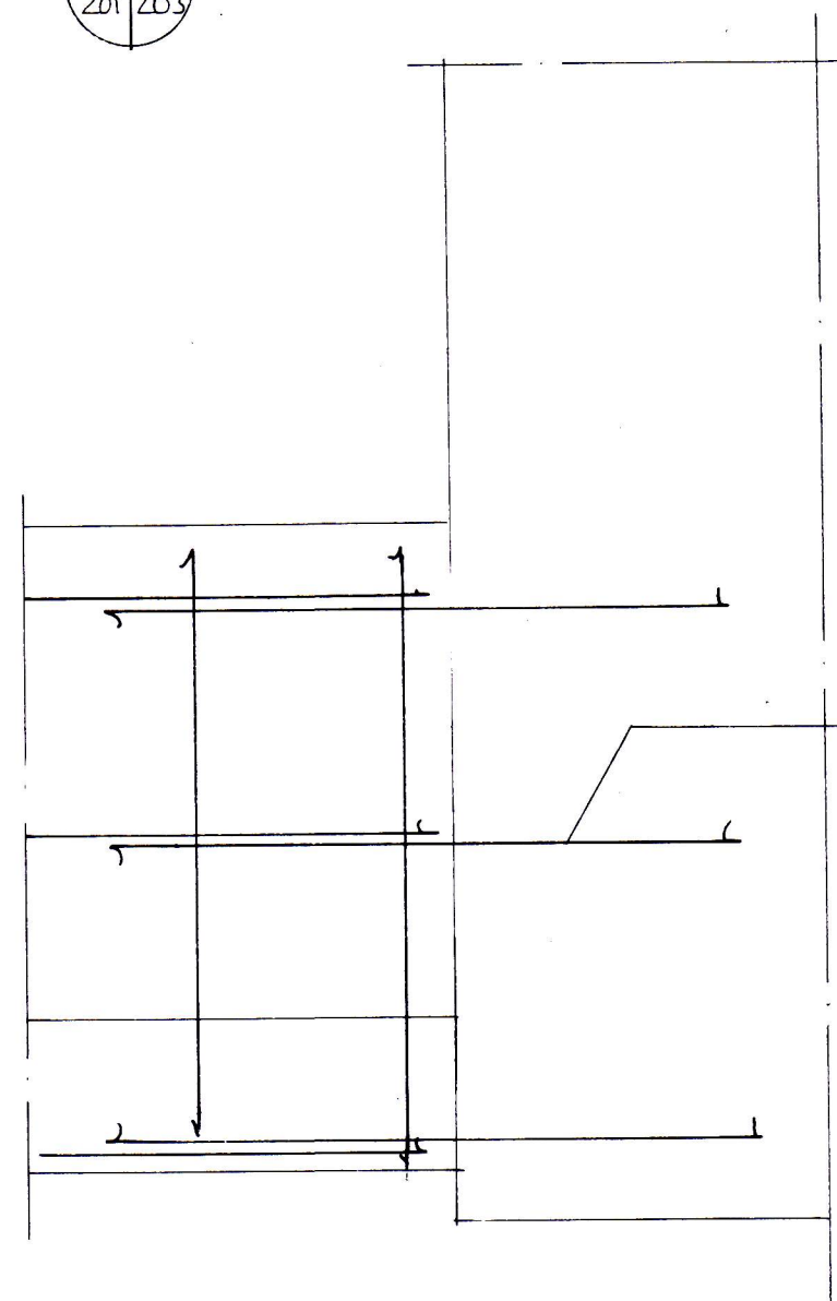
TENGING SÖKKLA M=1:10
