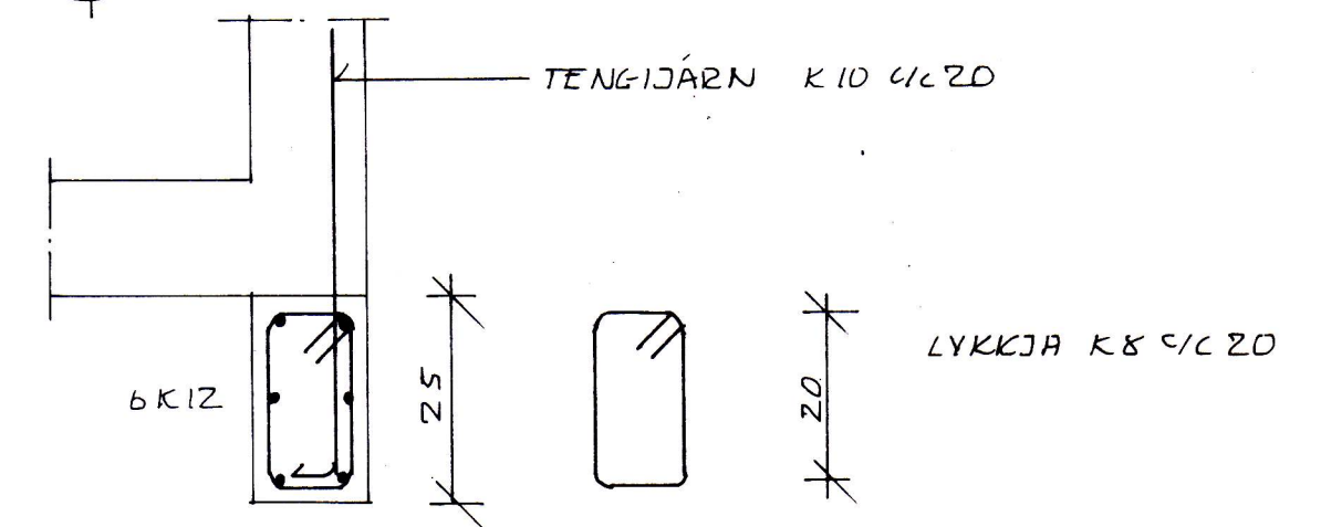
SÚLA S-2 M=1:20
