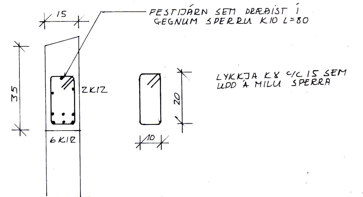
ÞÍTI B-1 M=1:10
