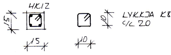
SÚLA S-1 M=1:20
