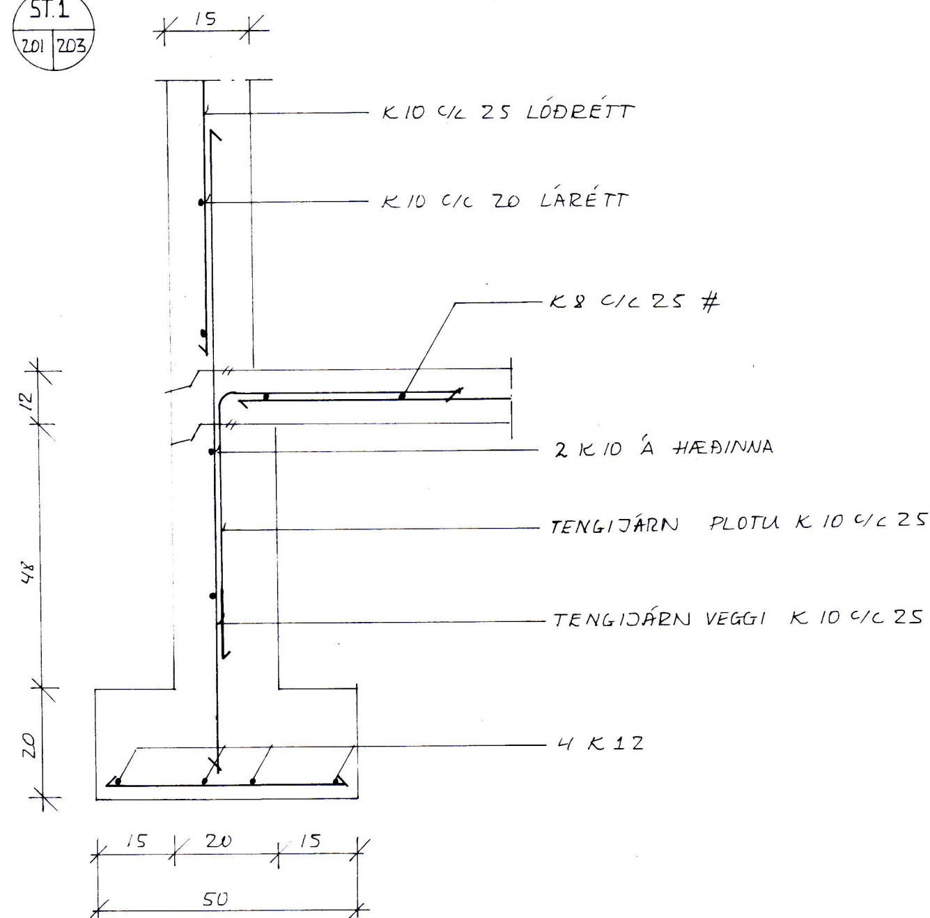
SNÍÐ Í SÖKKLA M=1:10
