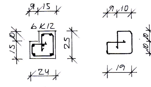
SÚLA S-2 M=1:20
