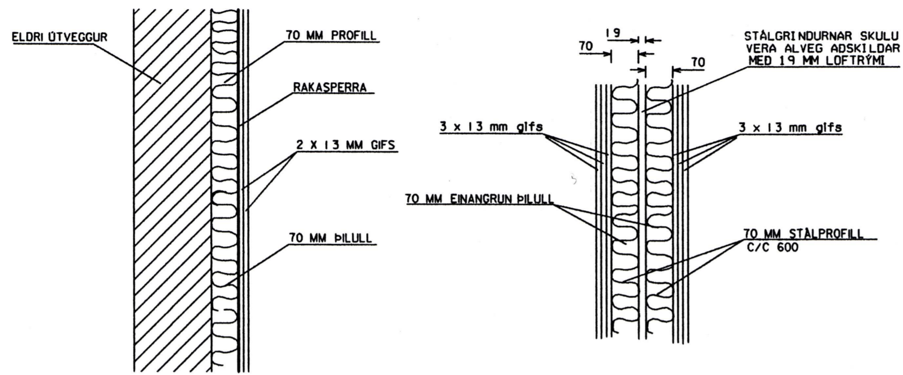
ÚTVEGGUR SNID B - B 1:10 SNID A - A 1:10
