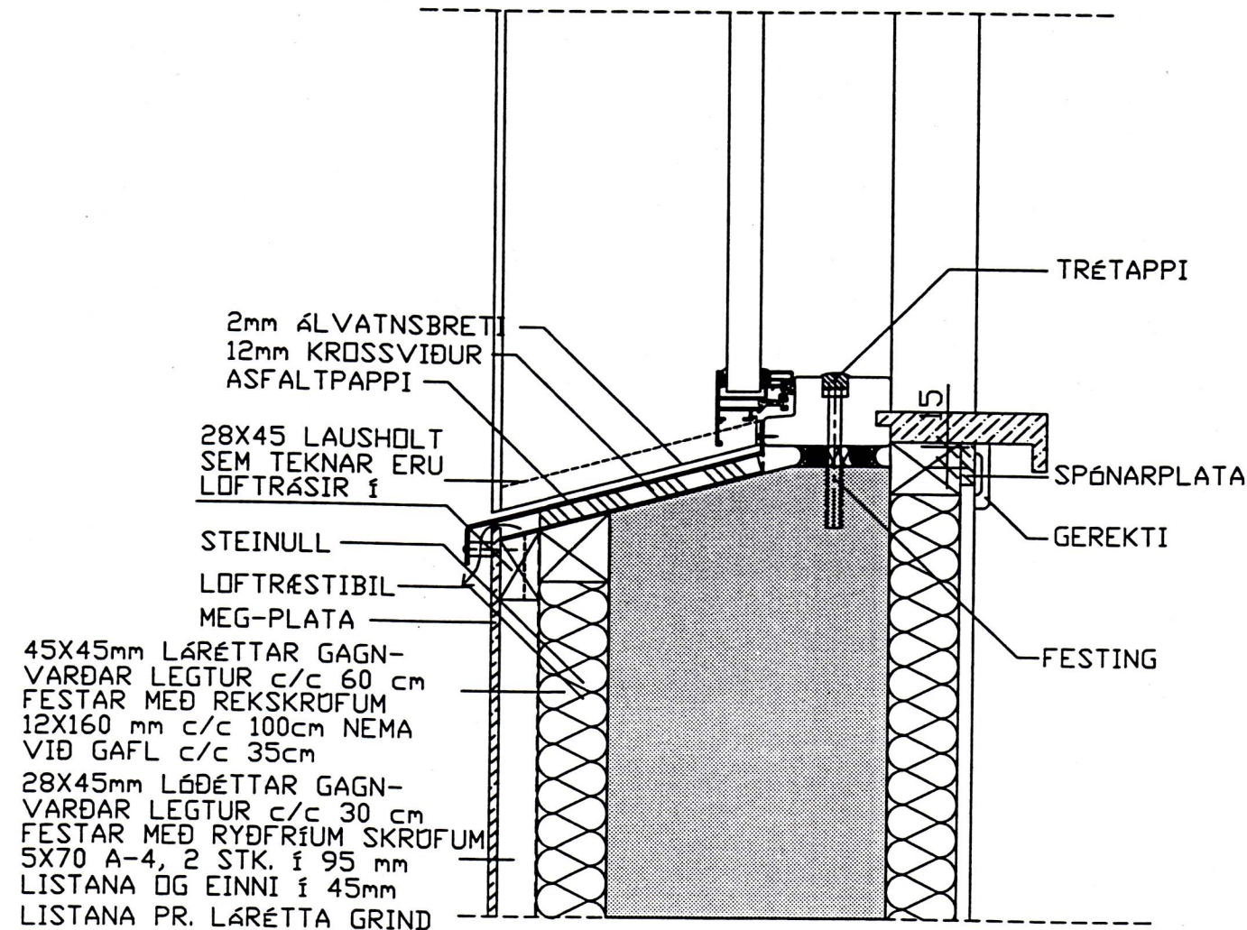
LÓÐRÉTT SNIÐ
