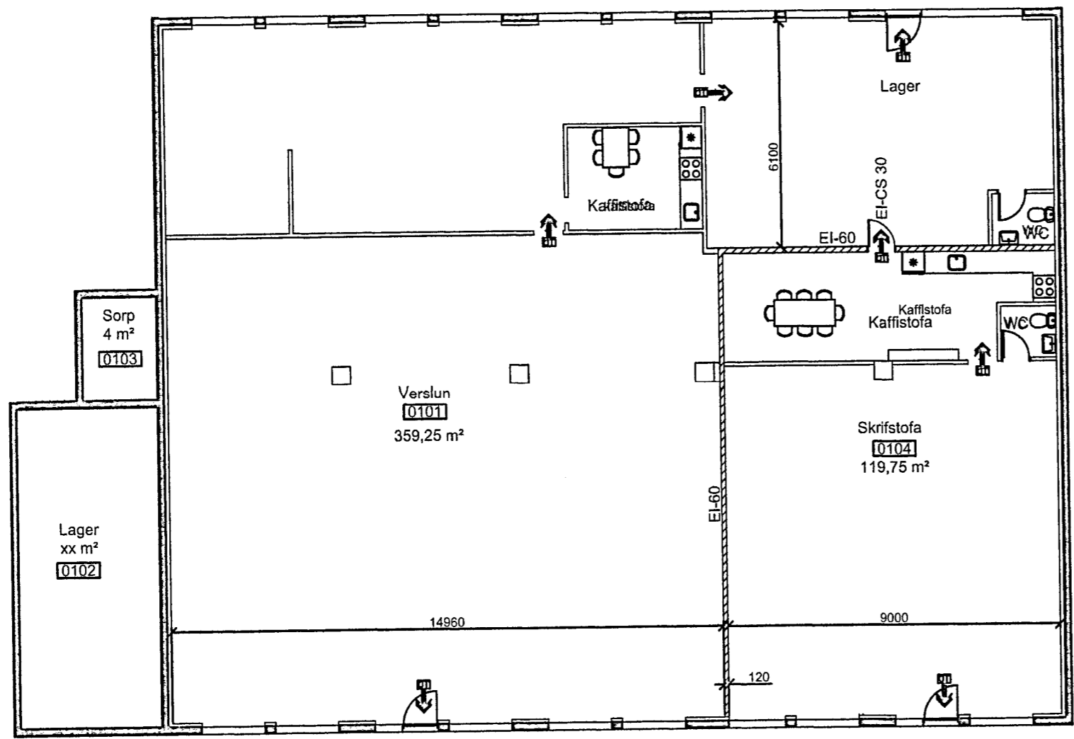
Grunnmynd eignaskipting
