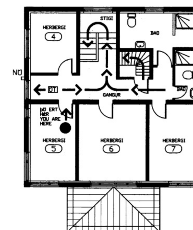
GRUNNMYND 2. HÆÐ
