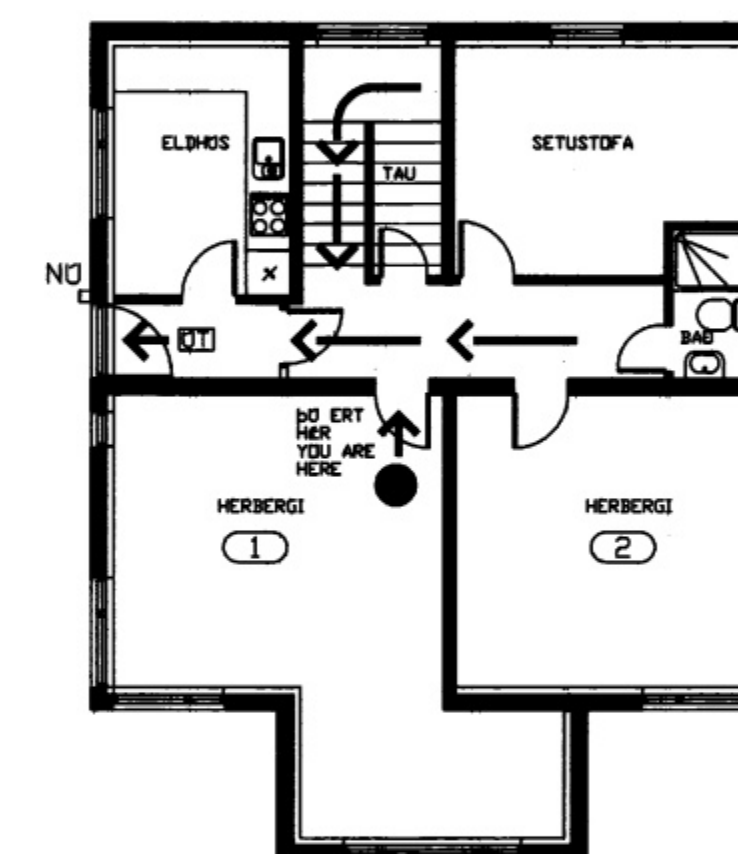
GRUNNMYND 1. HÆÐ
