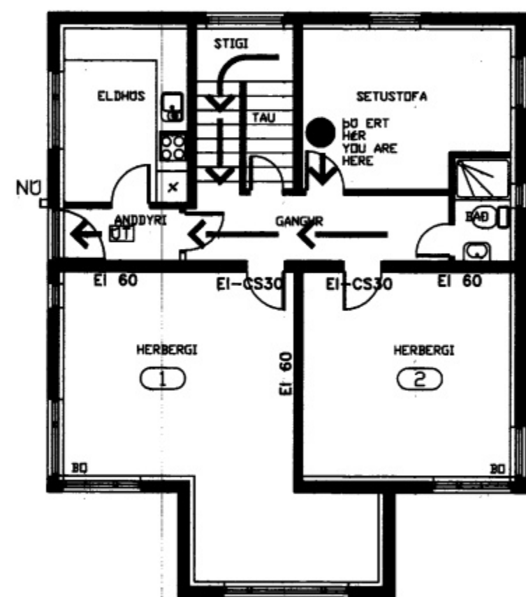
GRUNNMYND 1. HÆÐ
