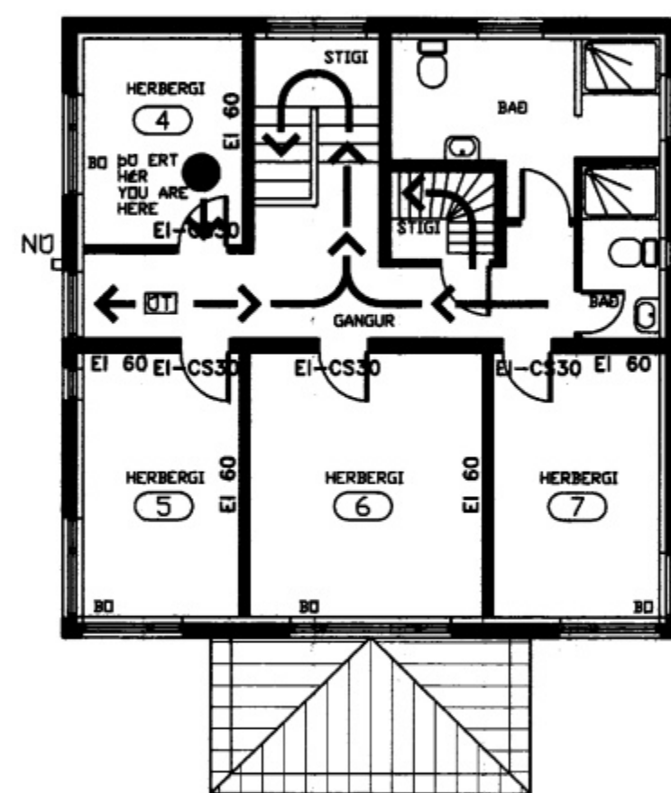
GRUNNMYND 2. HÆÐ
