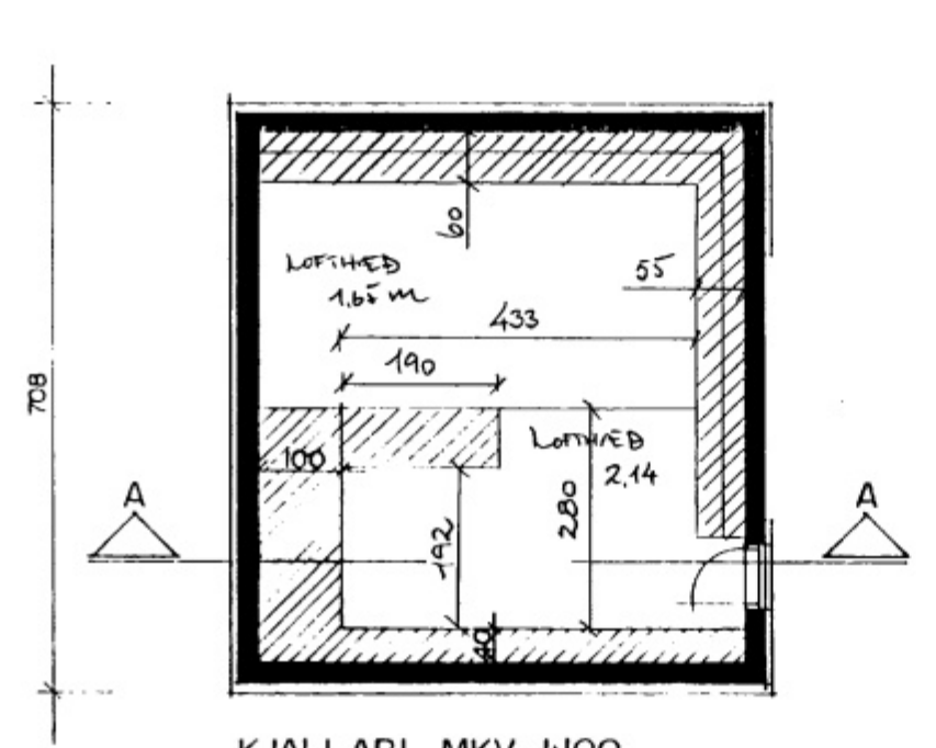
KJALLARI MKV. 1:100
