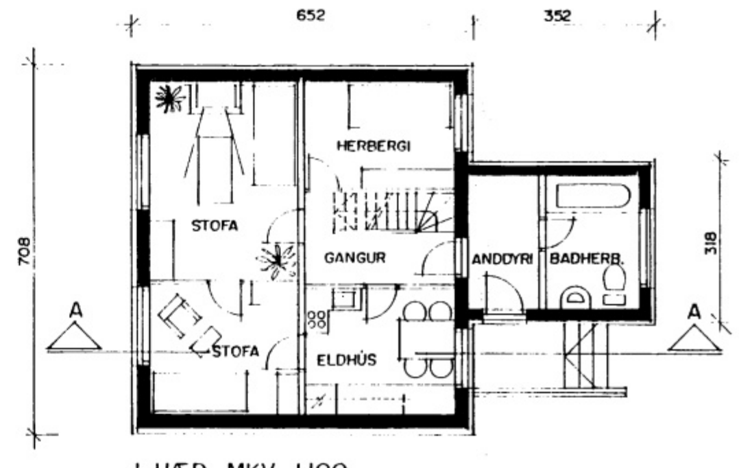
1. HÆÐ MKV. 1:100
