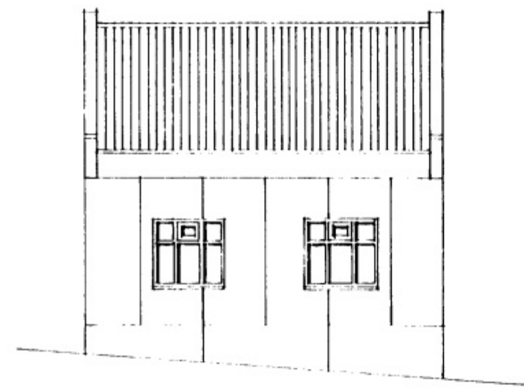
SUÐUR MKV. 1:100
