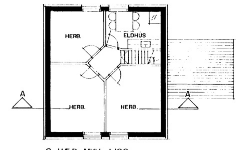
2. HÆÐ MKV. 1:100
