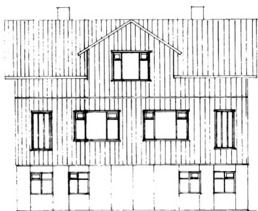
SÚÐURHLÍÐ MKV 1:100
