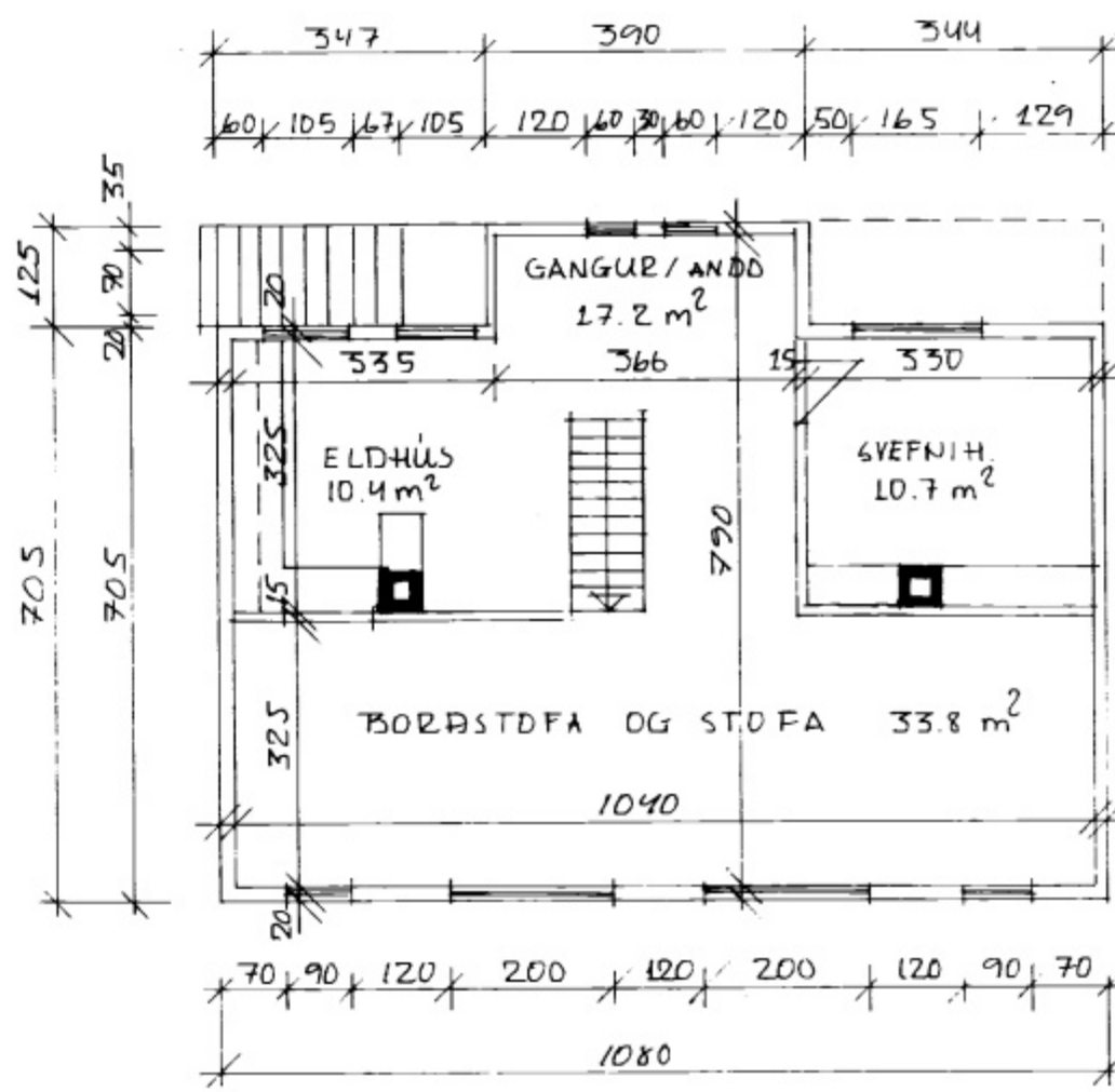
MIDHÆÐ MKV 1:100
