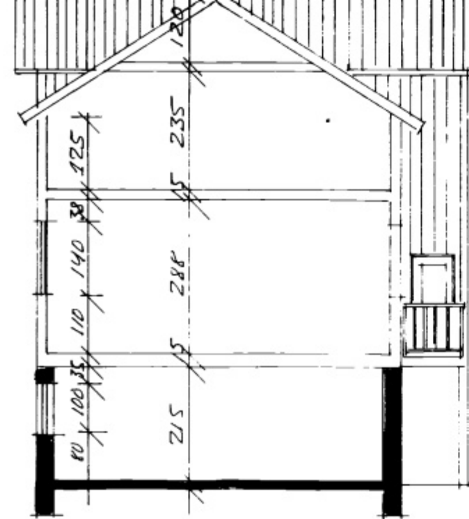
SNIB A-A MKV 1:100
