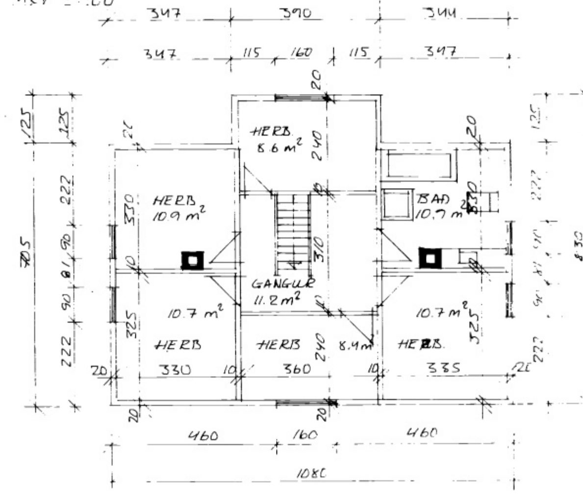
ÞAKHÆÐ MKV 1:100
