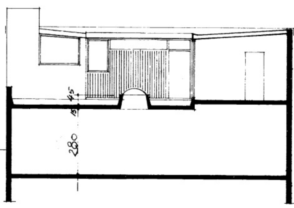
SKURÐMYND B-B
