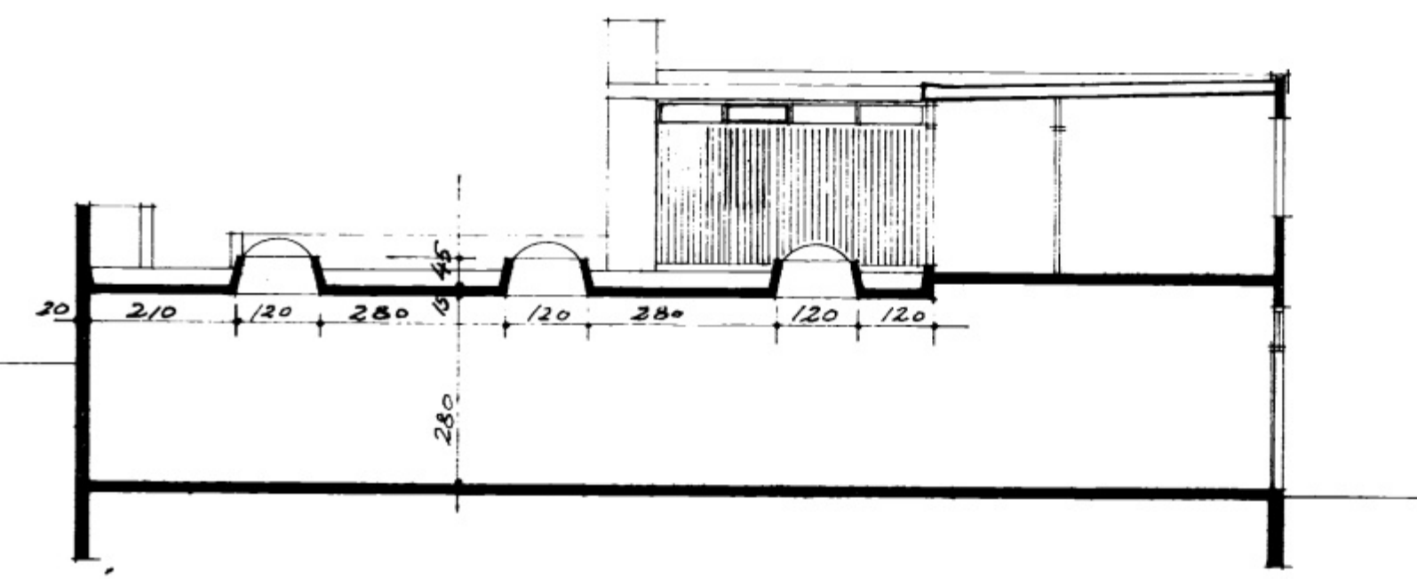
SKURÐMYND C-C ATH. ÖLFRÉKARI MÁLSETNING Á VINNUTEIKN. M:1:50
