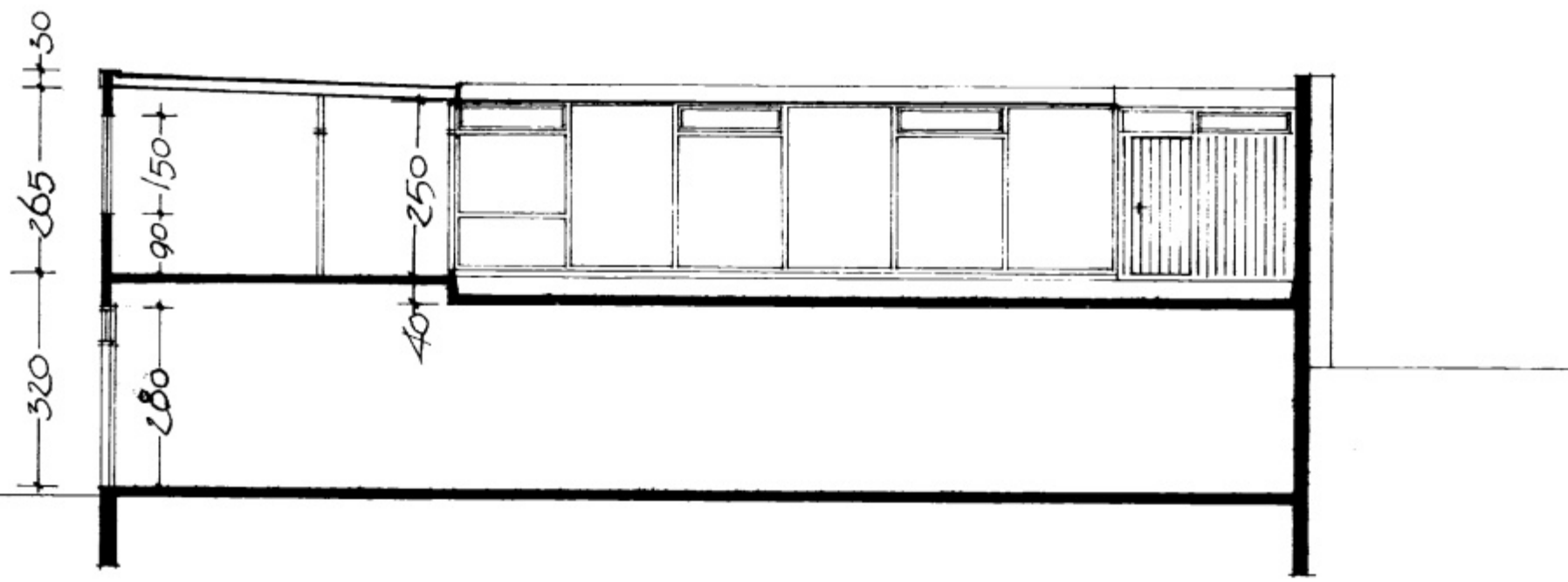
SKURÐMYND A-A
