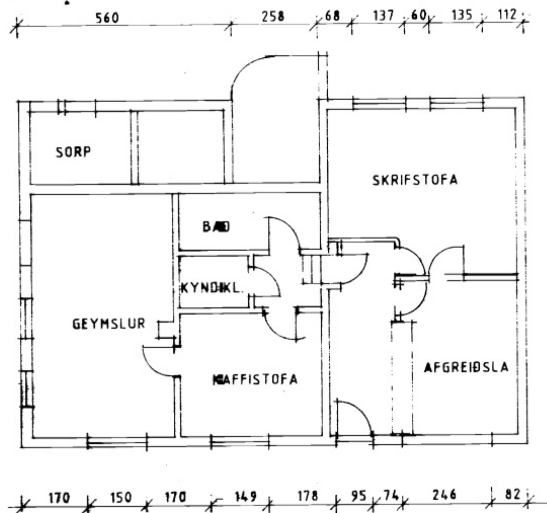
GRUNNMYND JARBÆÐ Mkv 1:100
