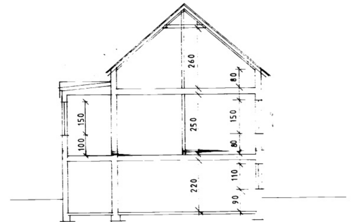
PVERSNIÐ Mkv 1:100
