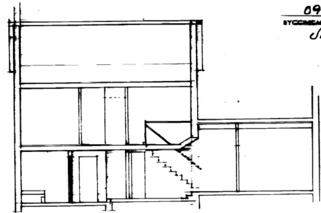
LANGSNID Mkv 1:100 A-A
