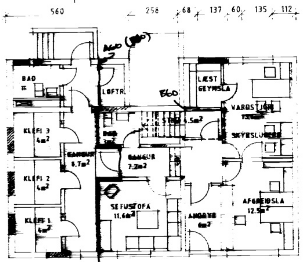
NORDURHLID
