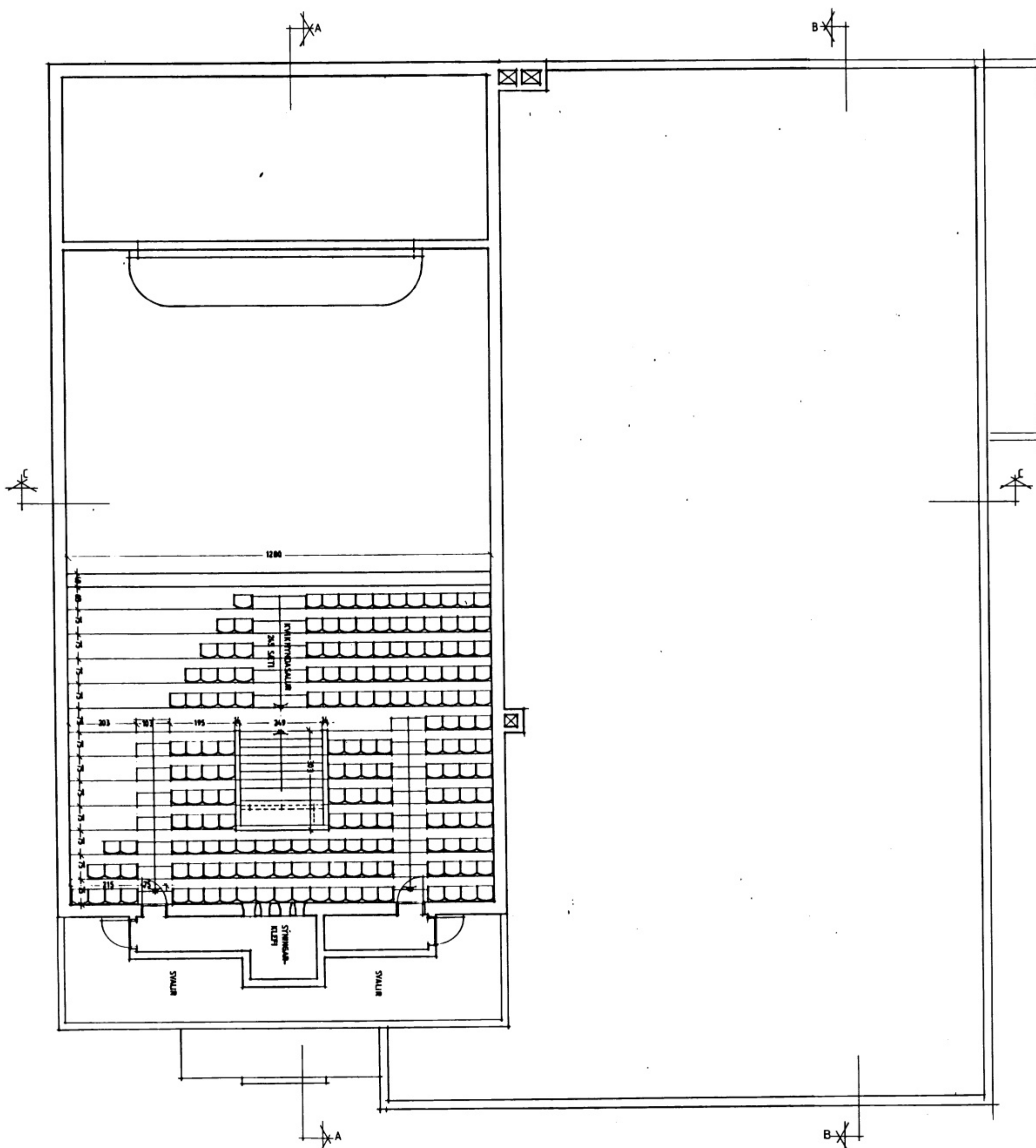
GRUNNMYND 3. HÆÐAR, MKV. 1:100, UPPMÆLING
