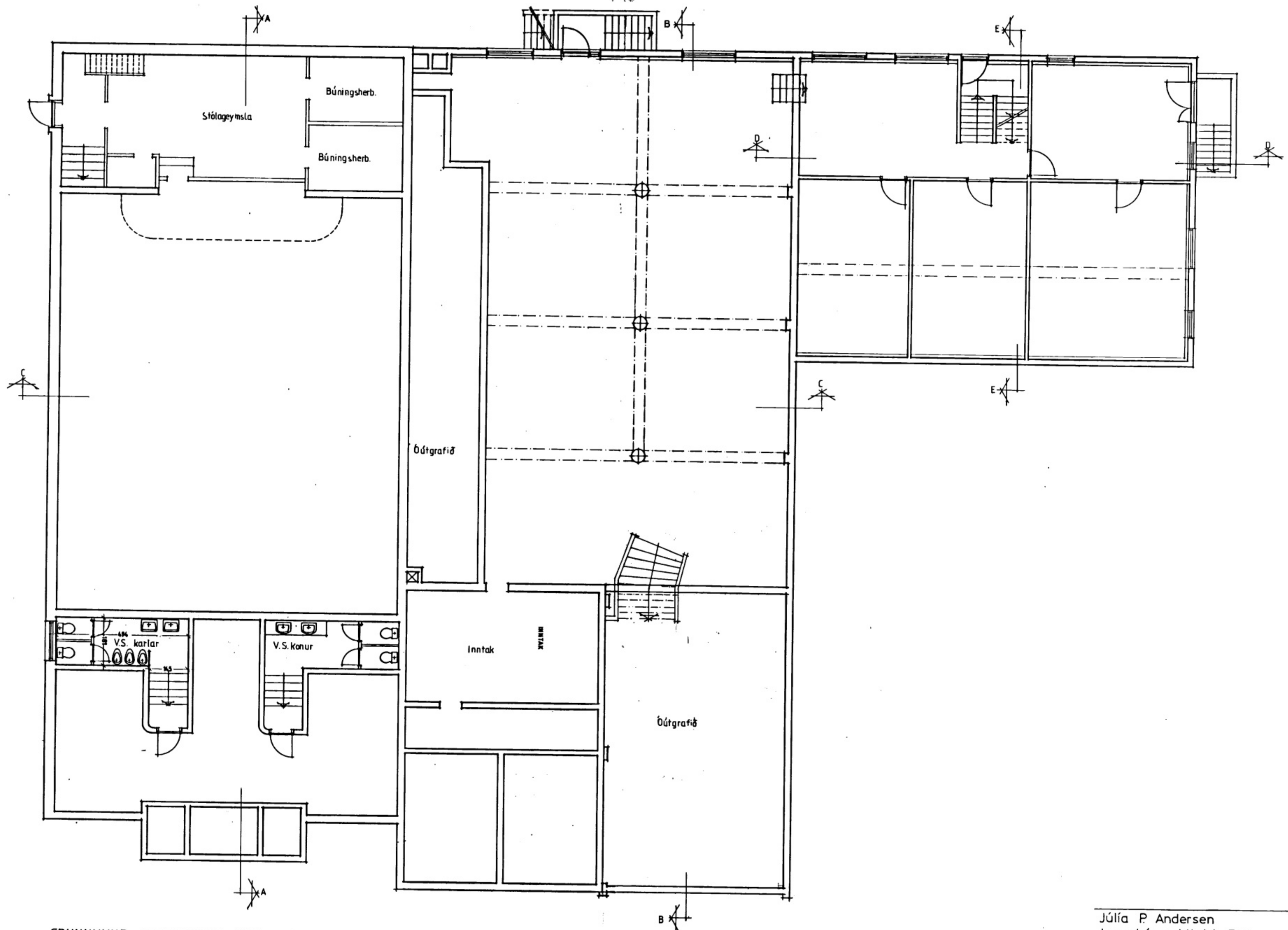
GRUNNMYND GRUNNHÆÐAR, MKV. 1:100, UPPMÆLING.
