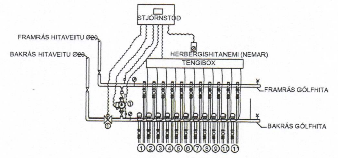
TENGRIND GÓLFHITA VESTURENDI 11 STÚTAR
