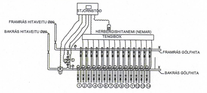
TENGRIND GÓLFHITA MIÐJA 14 STÚTAR
