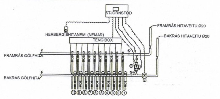
TENGRIND GÓLFHITA AUSTURENDI 10 STÚTAR
