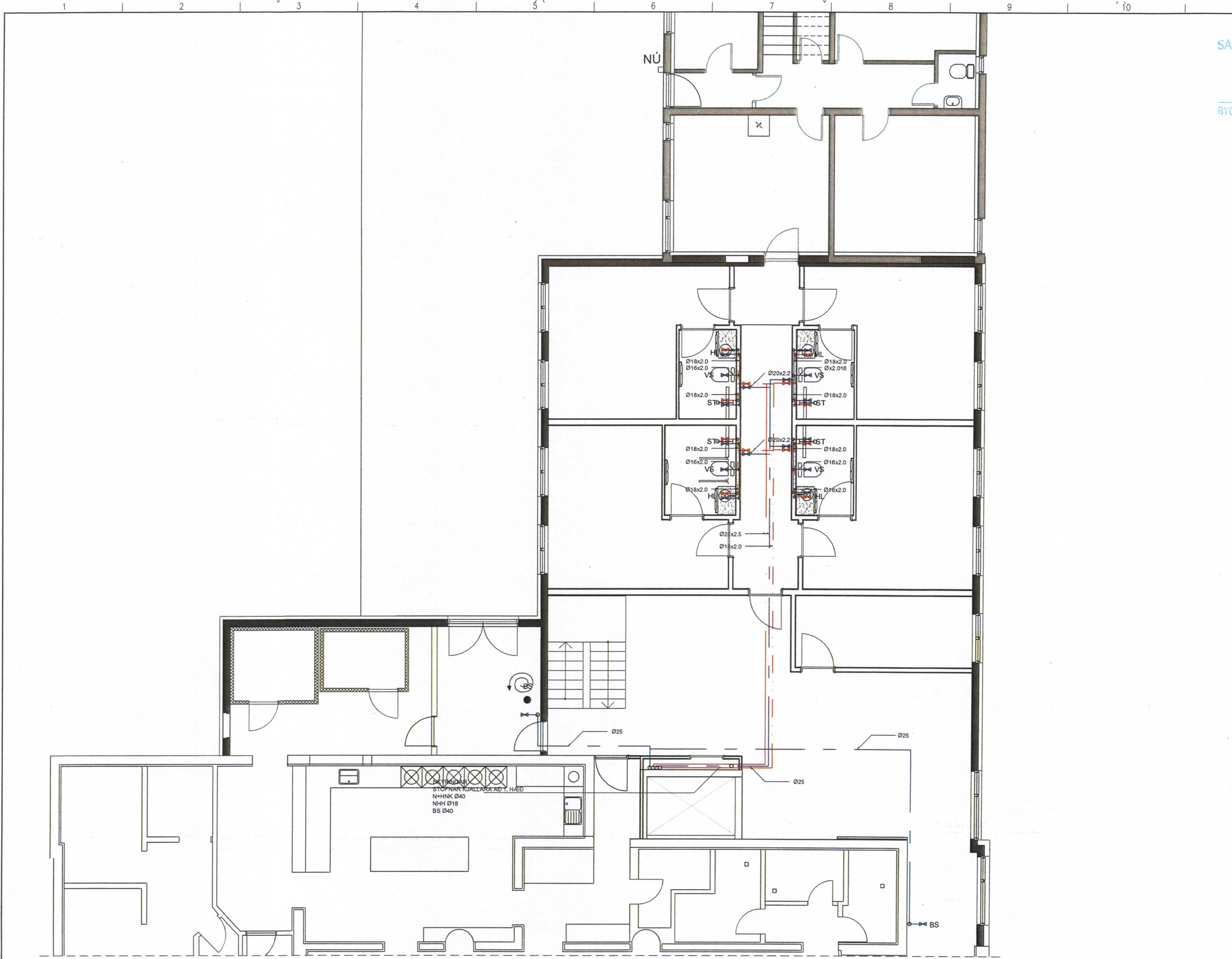
GRUNNMYND 1. HÆÐ VATNSLAGNIR M=1:50
