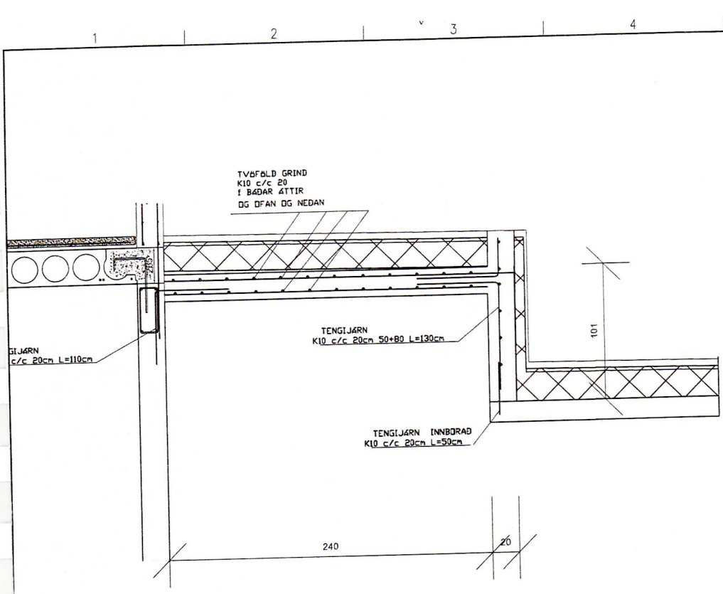
Burðarvirki 1:20
