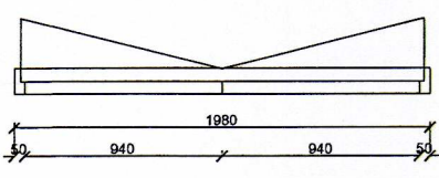
HURD H-1 1 STK. M=1:20 (NORDURHURD 1.HÆÐ VID FRYSTA)
