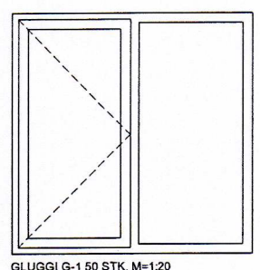
GLUGGI G-1 50 STK. M=1:20
