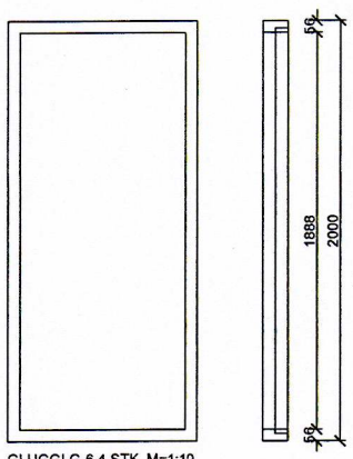
GLUGGI G-6 4 STK. M=1:10
