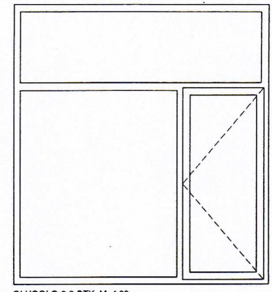
GLUGGI G-3 3 STK. M=1:20
