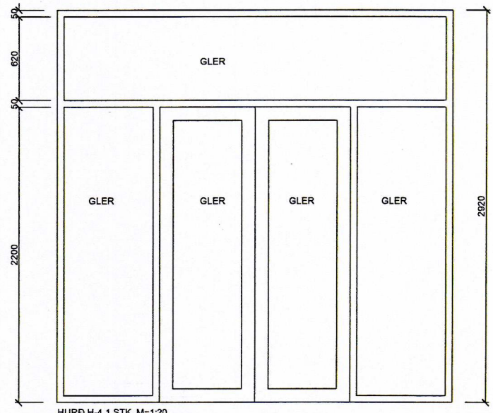
HURD H-4 1 STK. M=1:20 (ADALINNGANGUR AD SUNNAN)
