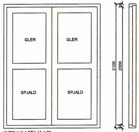
HURD H-2 1 STK. M=1:20 (VESTURHURD KJALLARI GEYMSLA)
