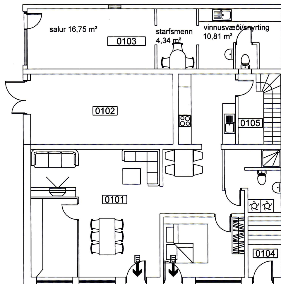
grunnmynd neðri hæð, mkv 1:100
