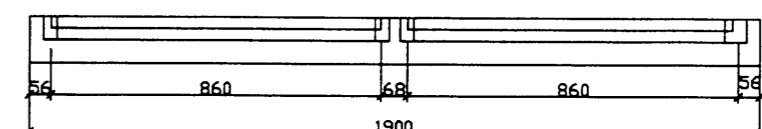
GLUGGI G-5 M=110 1 STK
