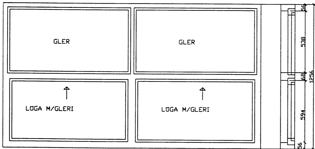
ÞTÍHURÐ H-2 M=110 2 STK
