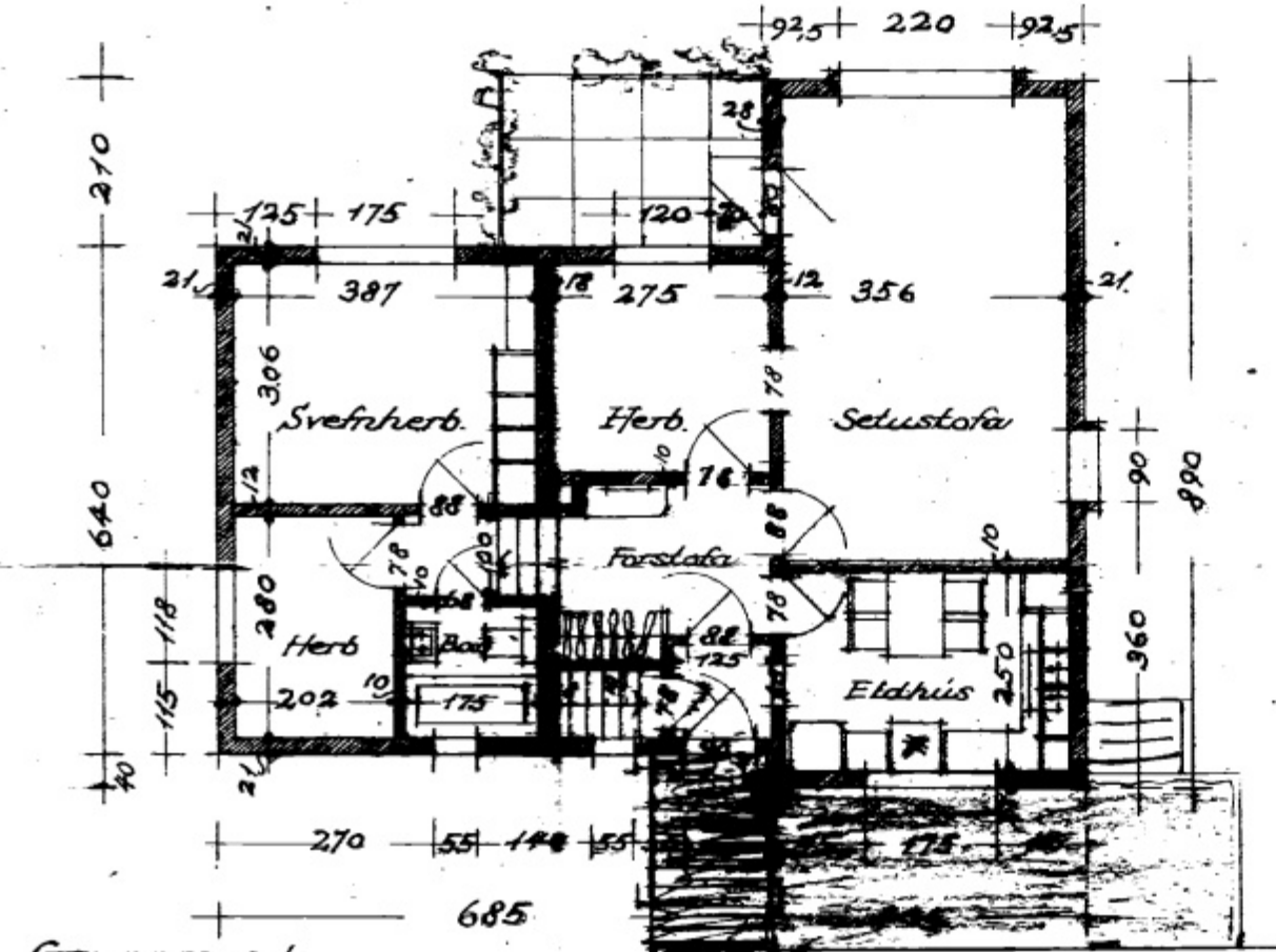
Grunnmynd
