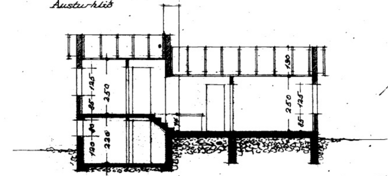
pólanskurður
