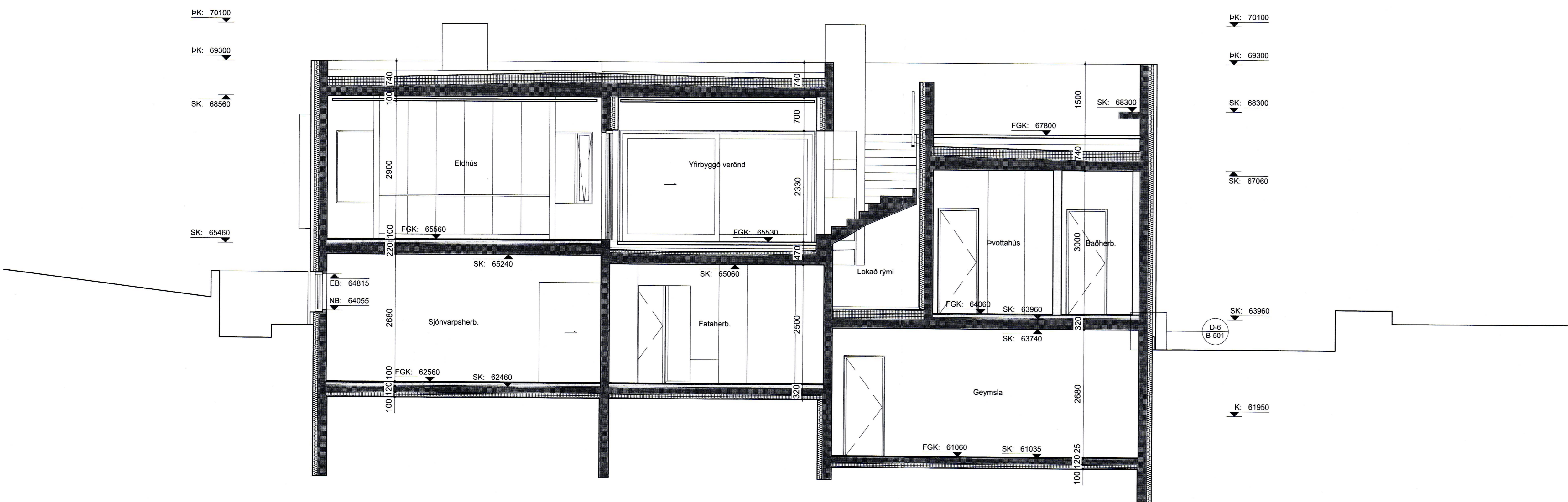
Sneiðing F-F mkv: 1:50
