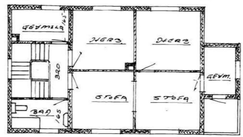
2. HÆÐ
