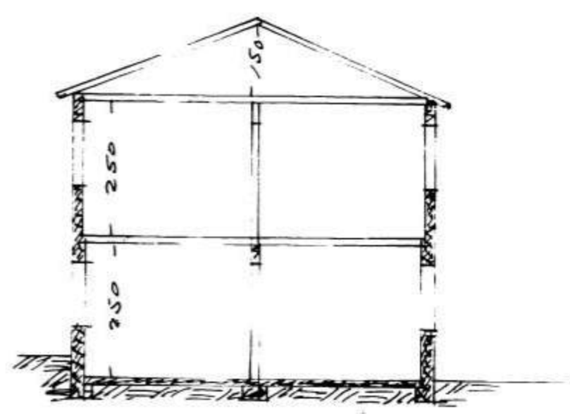
SKURÐUR
