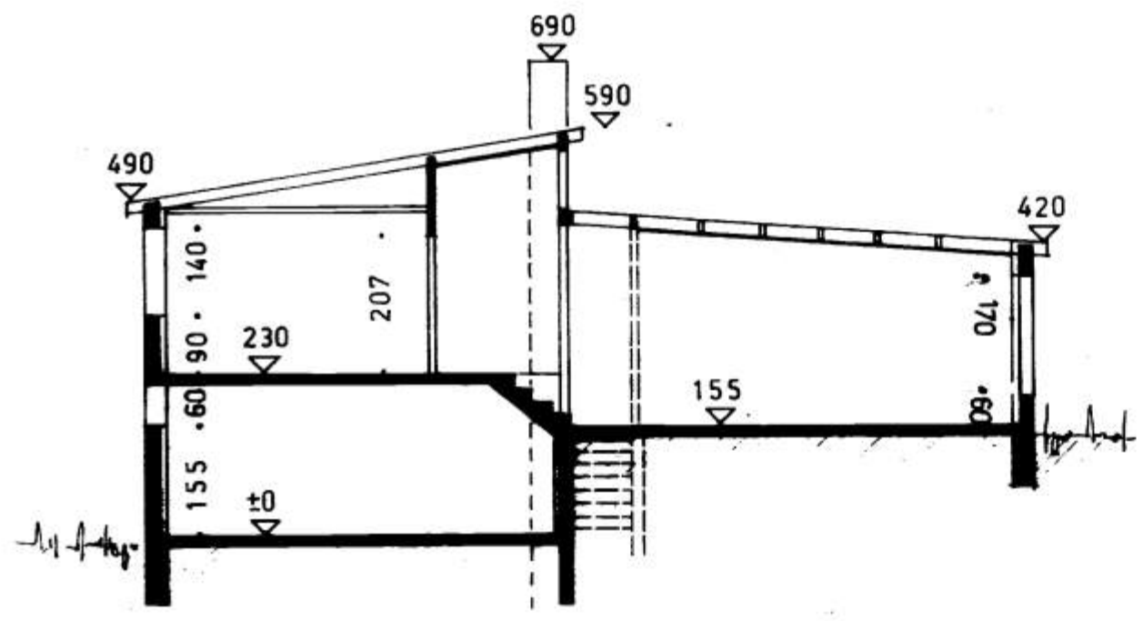
sneiðing a-a
