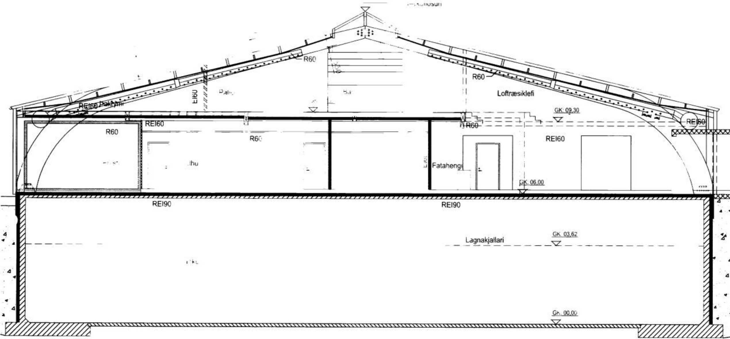
SNID A-A
