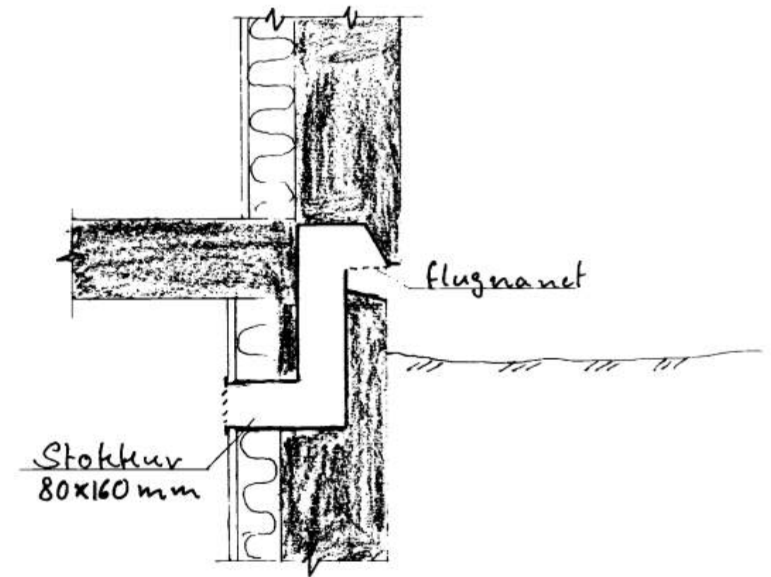
Snid A-A
