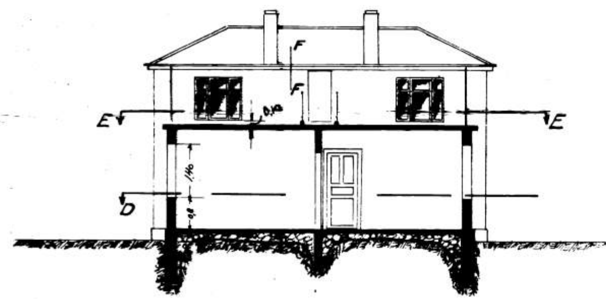
Snið B-B
