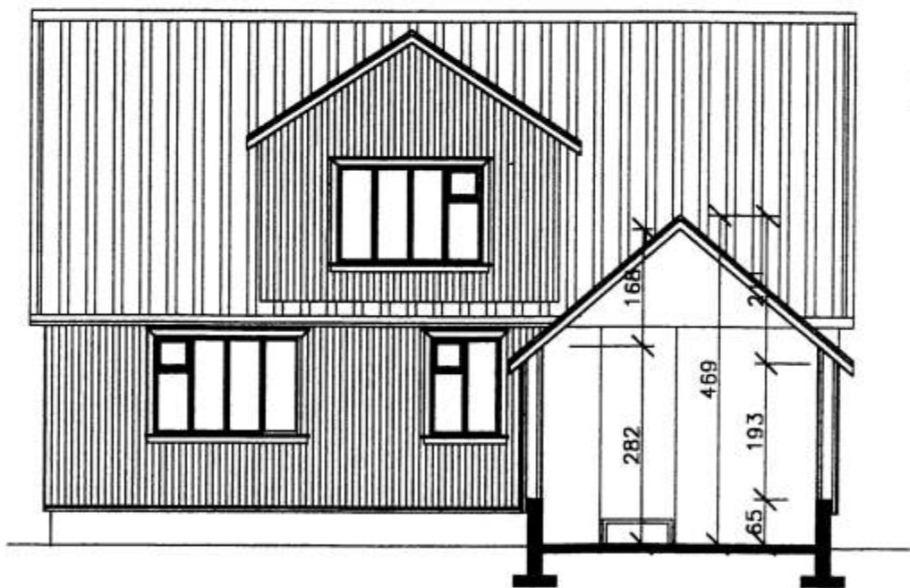
SNİÐ B-B Í GEGNUM BÍLSKÚR M=1:100
