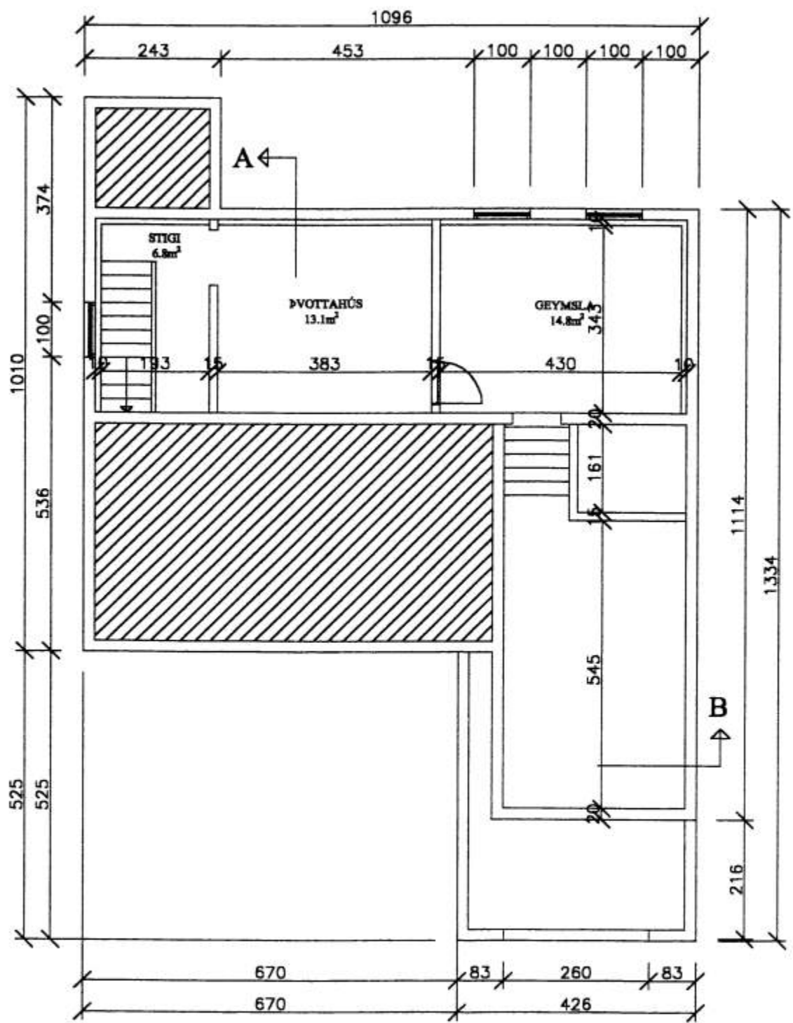
GRUNNMYND KJALLARI M=1:100
