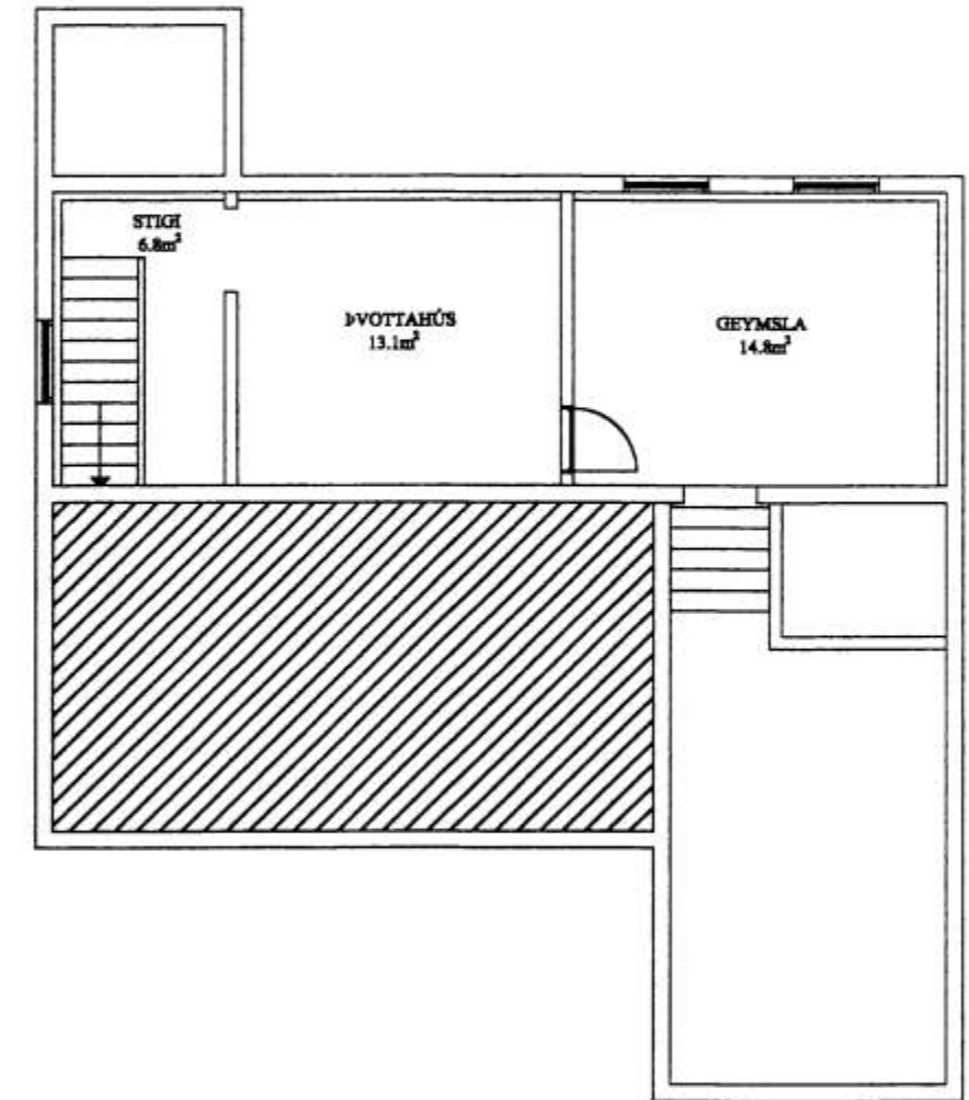
GRUNNMYND KJALLARI M=1:100
