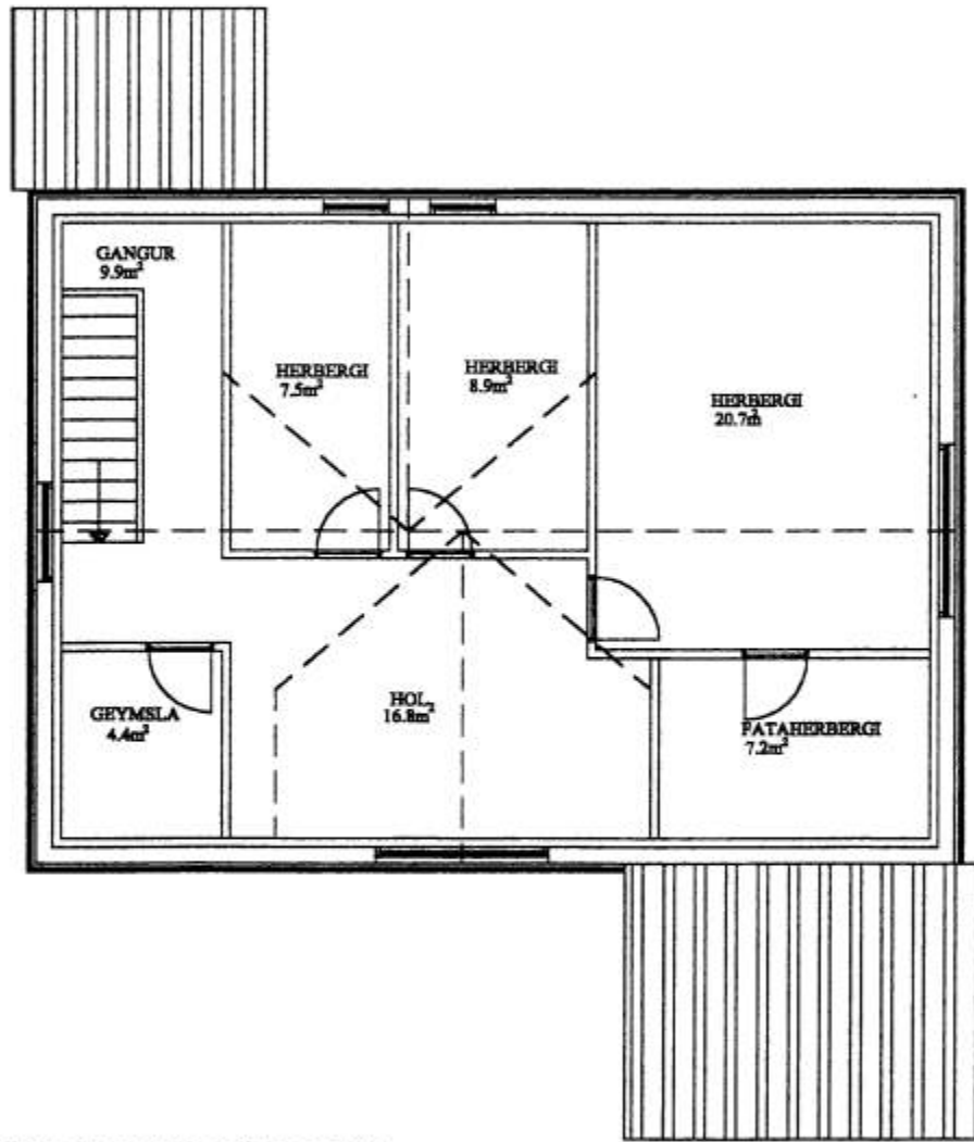
GRUNNMYND RIS M=1:100
