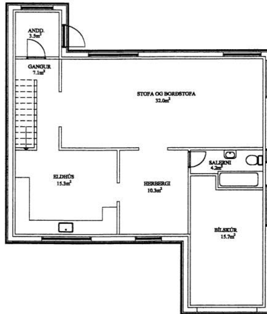
GRUNNMYND 1 HÆÐ M=1:100
