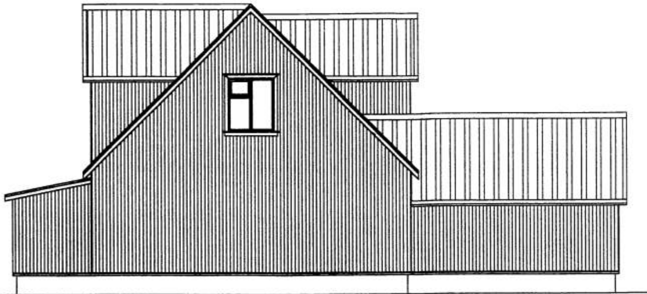
AUSTURHLIÐ M=1:100
