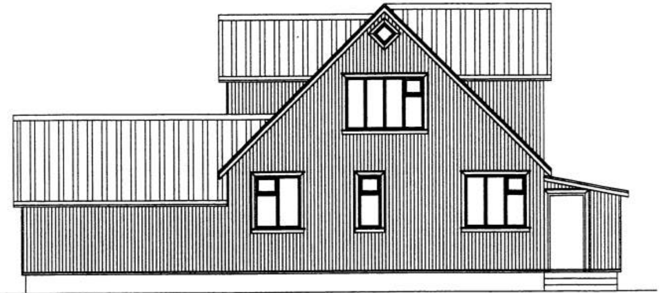
VESTURHLIÐ M=1:100
