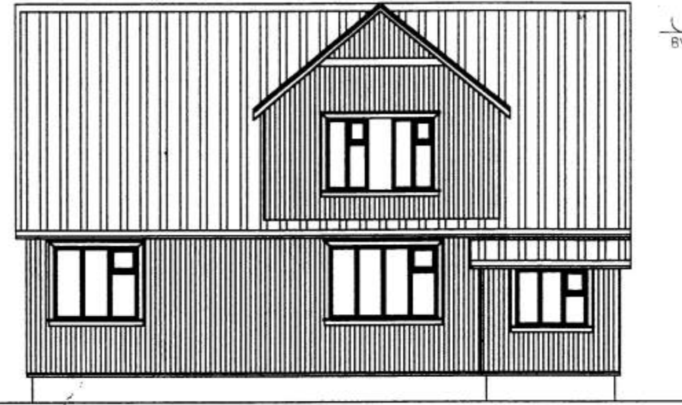
SUÐURHLIÐ M=1:100
