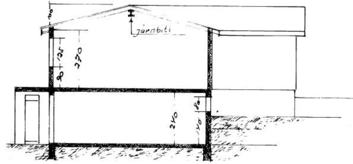
SKURÐUR A-A
