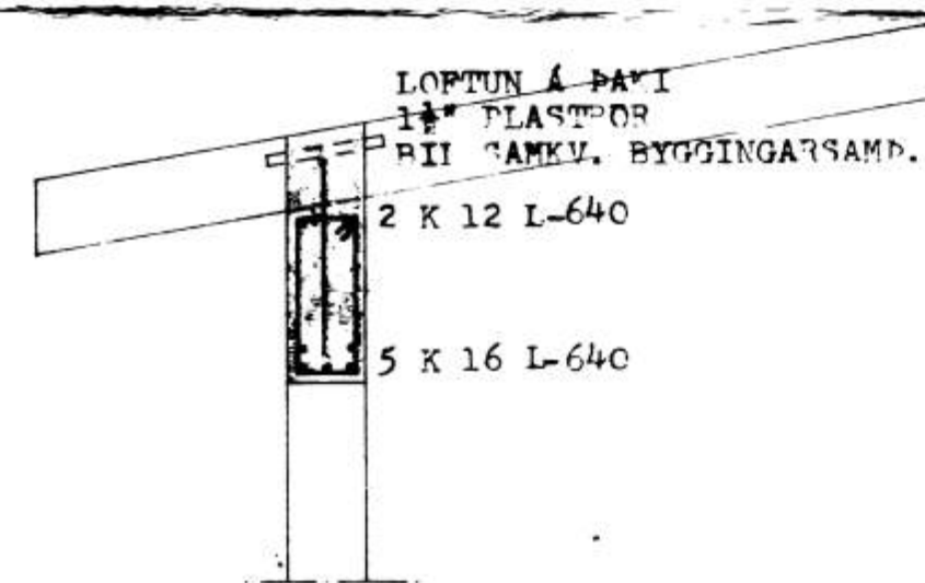
SNID - E 1:20
