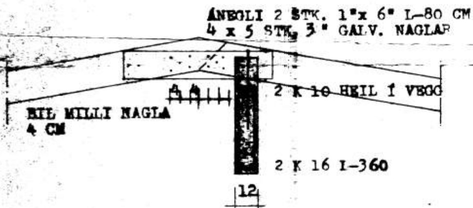
SNID - C 1:20
