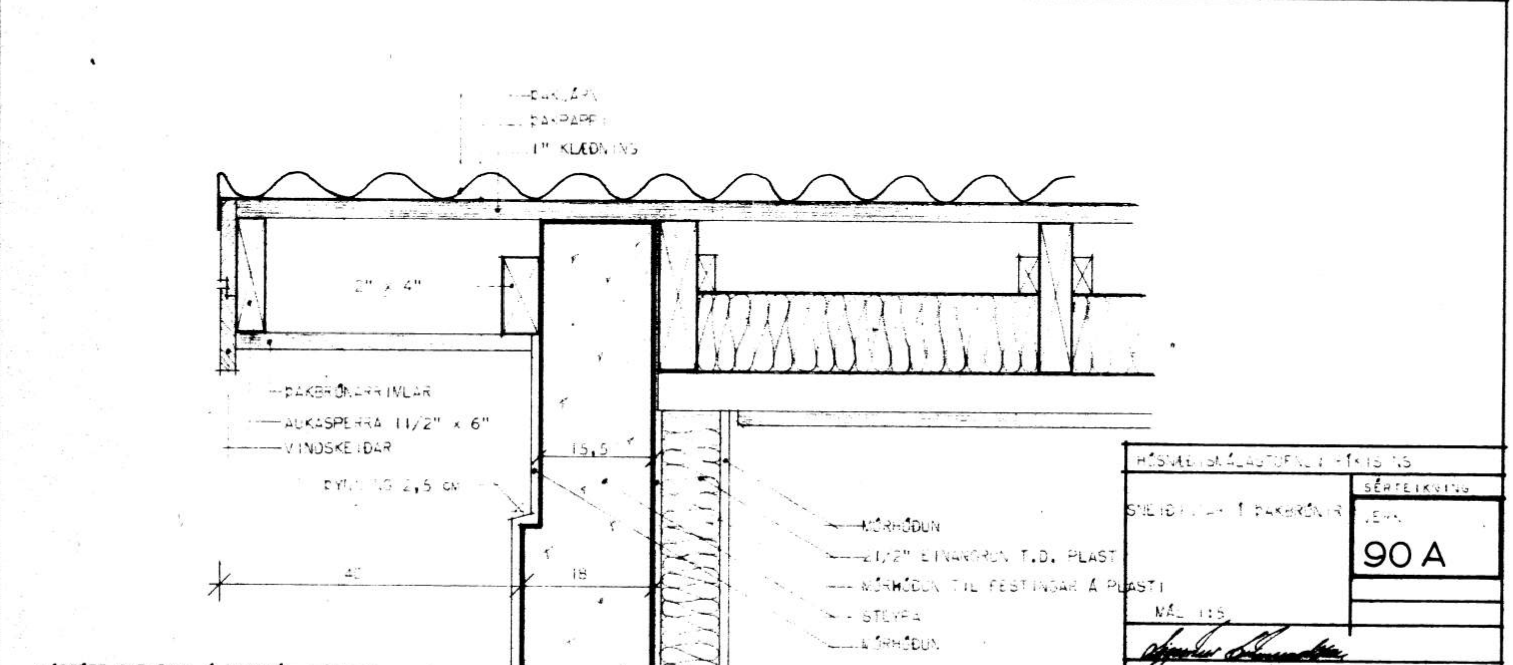
LÖÐRÉTT SNEIÐING Í DAKBRUNN AÐ DARI
