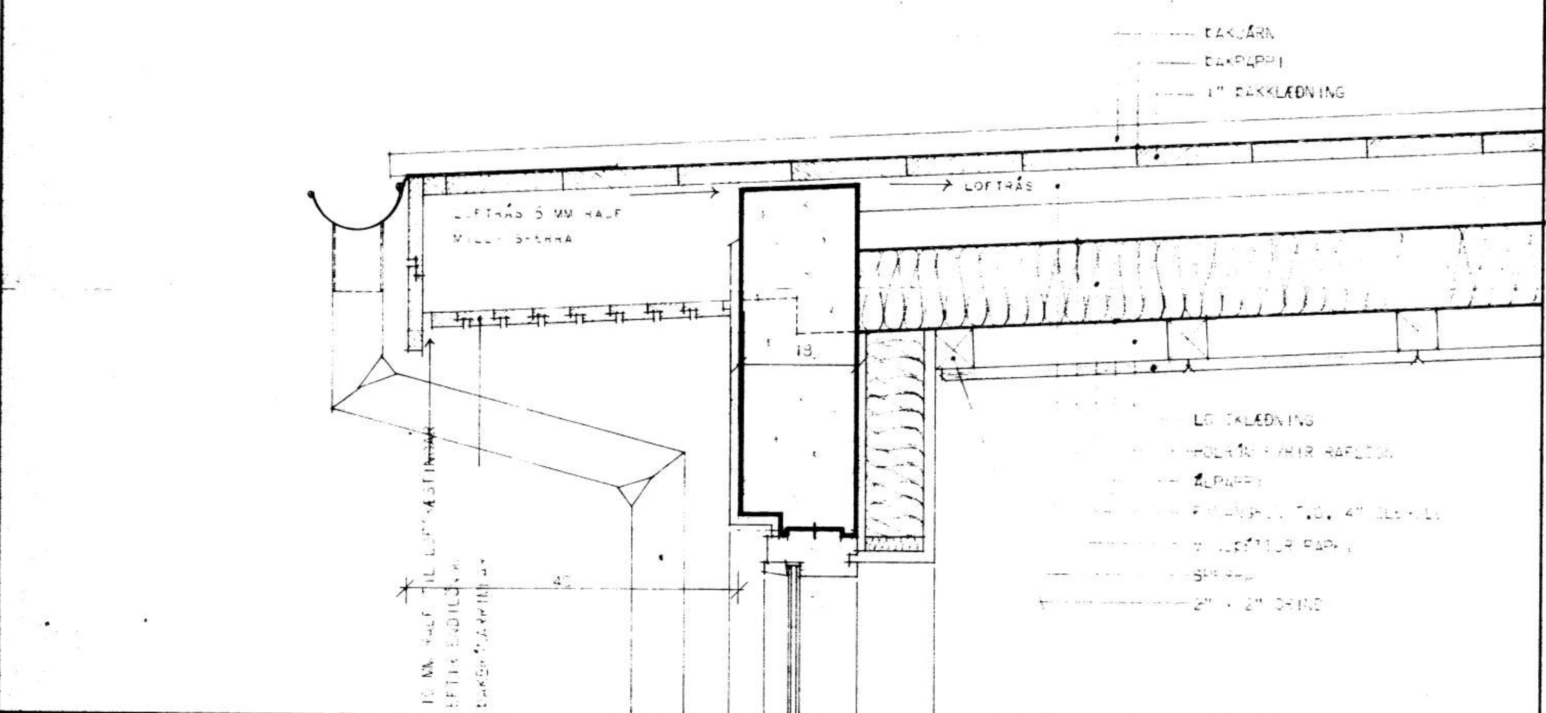
LÖÐRÉTT SNEIÐING Í DAKBRUNN AD FRYMAN
