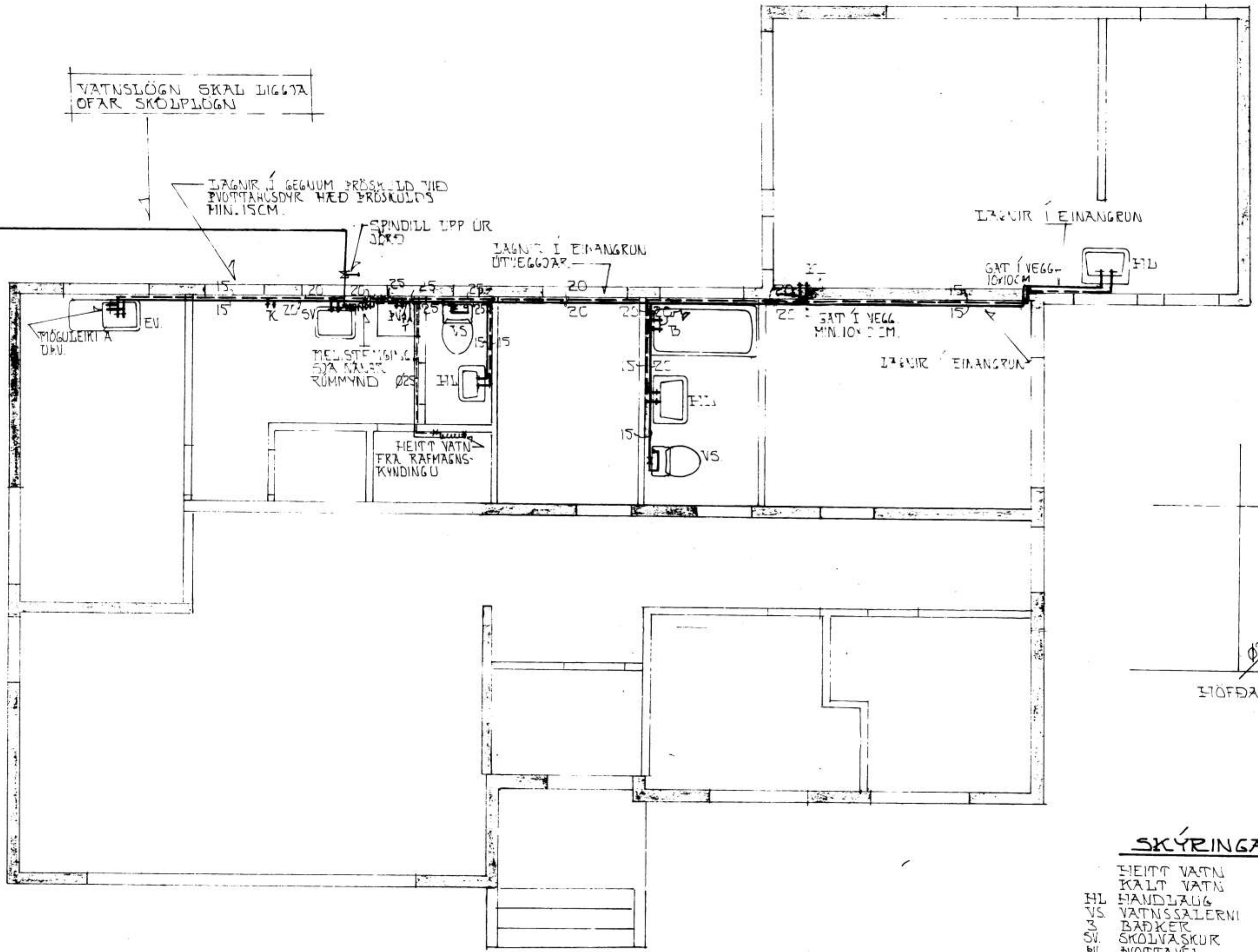
GRUNNMYND 1:50
