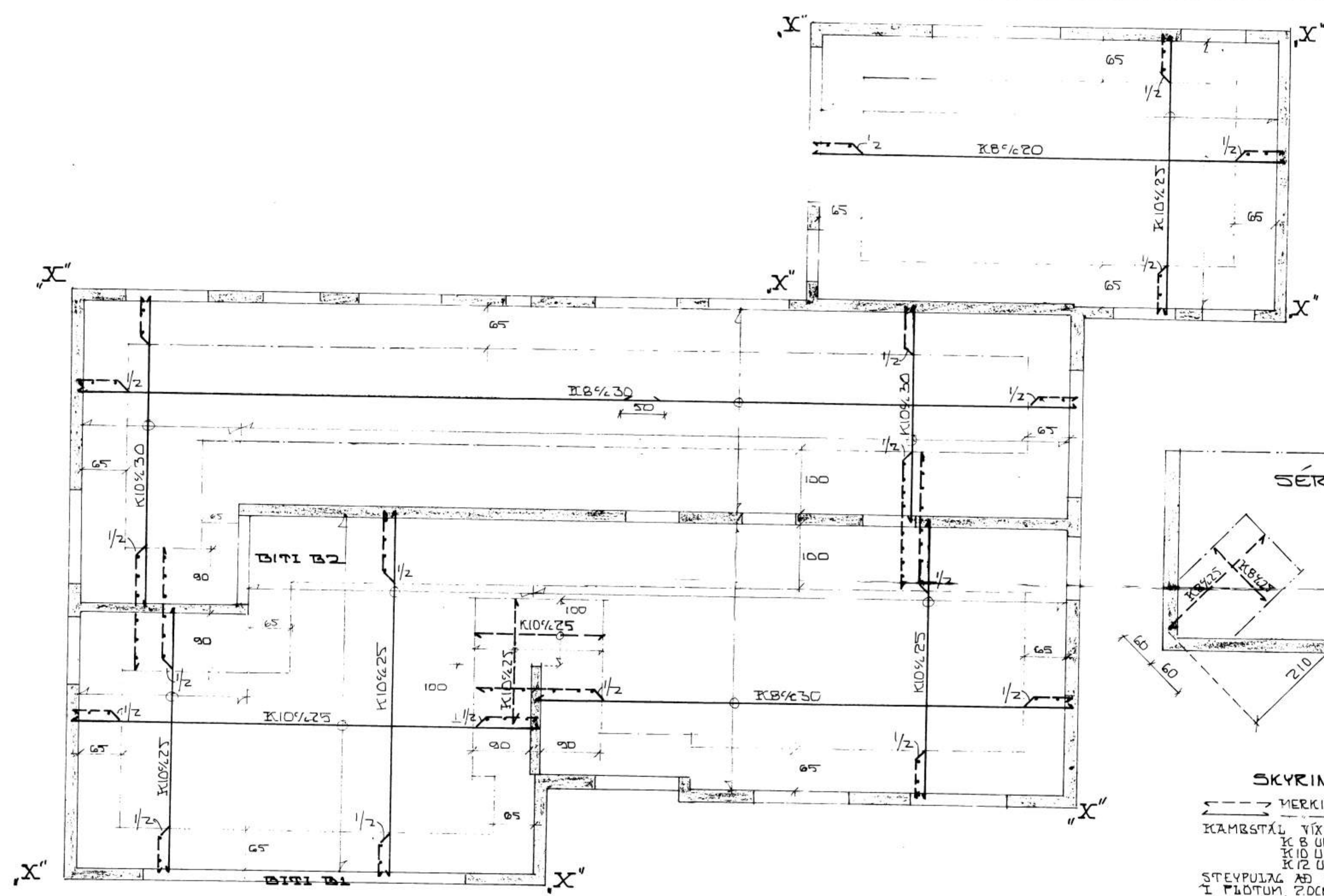
GRUNNMYND 1:50
