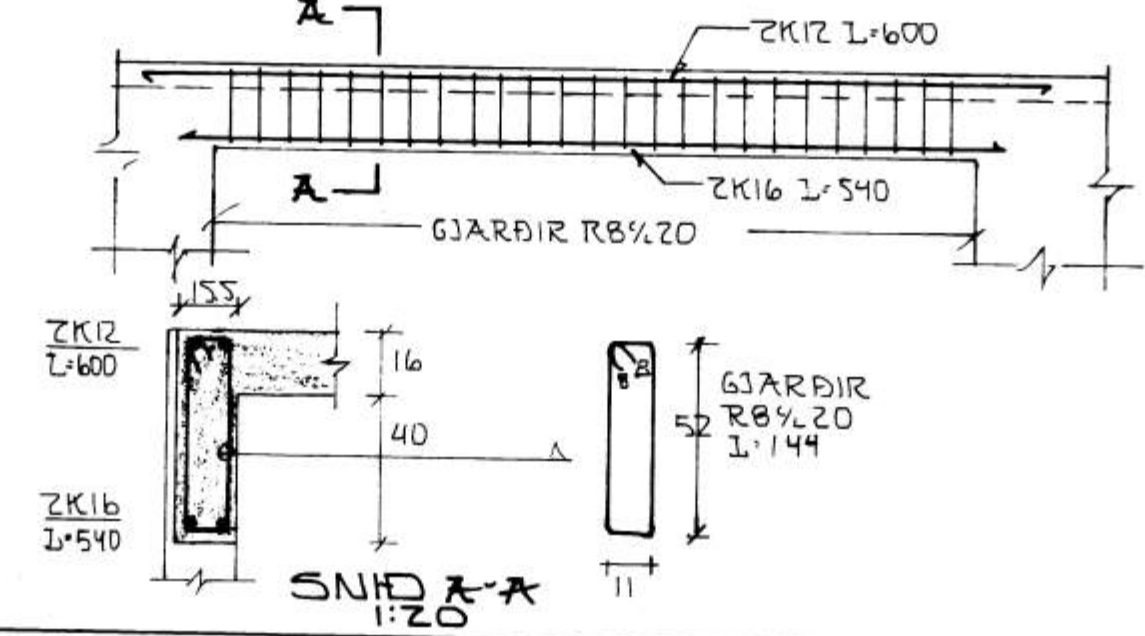
JÄRN Í BITA B1 1:50
