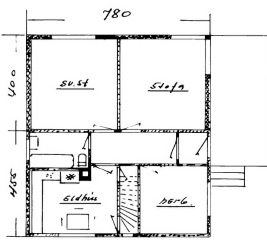
GRUNNFLÖTUR
