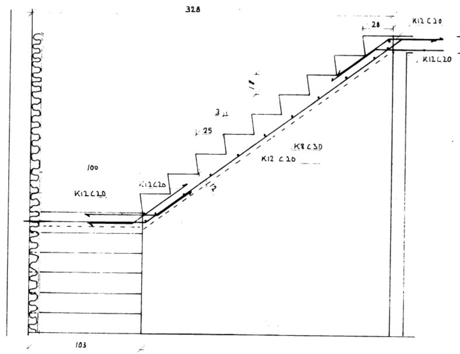
TRÖPPUR MKV 1:20
