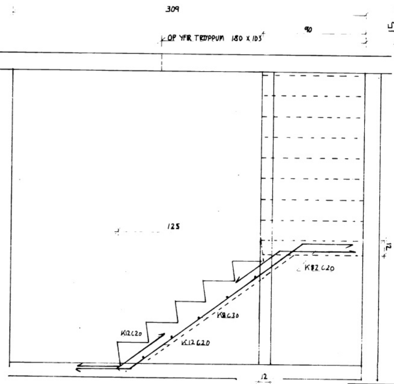
TRÖPPUR MKV 1:20
