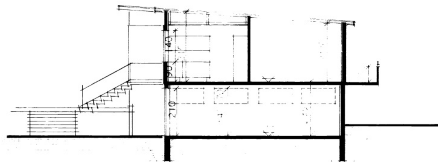
SNITUR A-D
