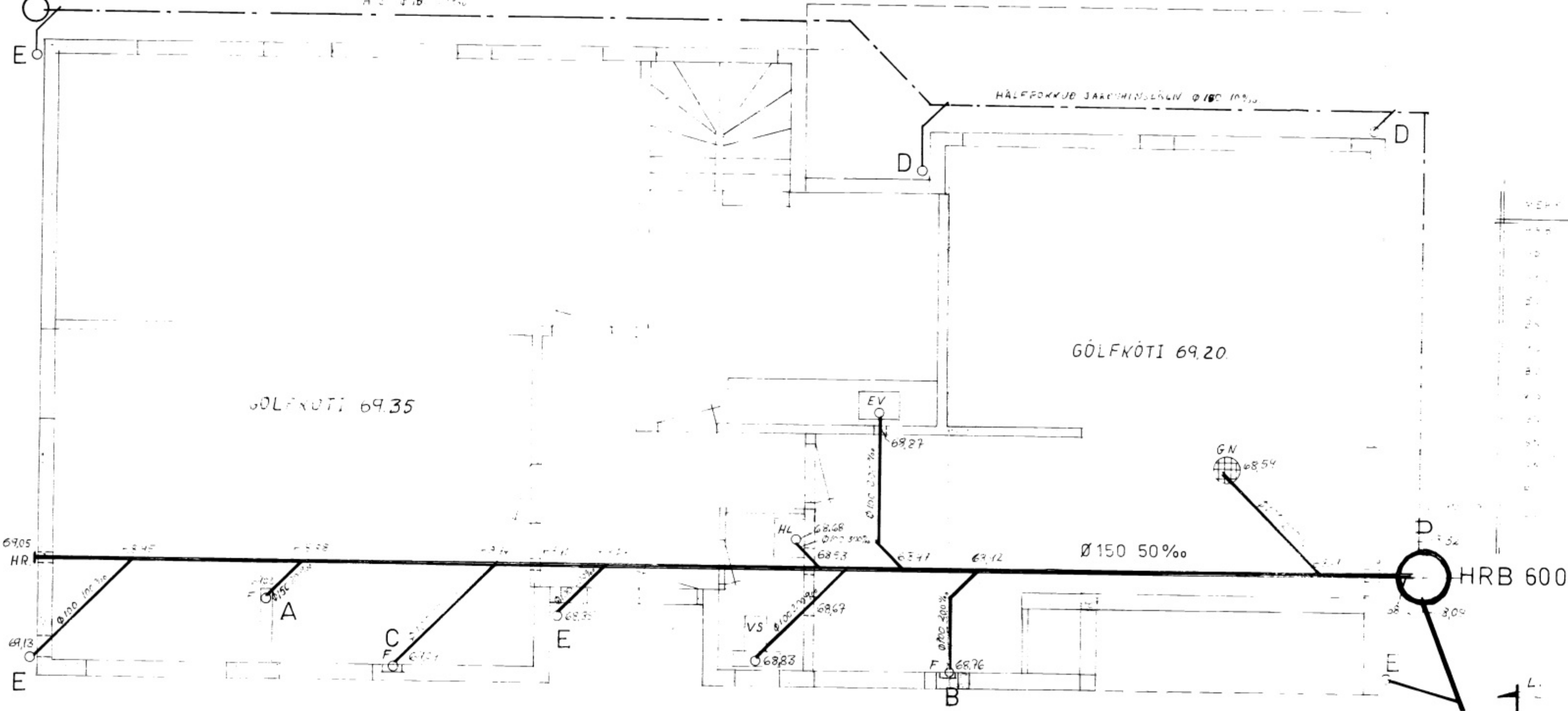
GRUNNMYND N-HÆÐAR M 1:50
