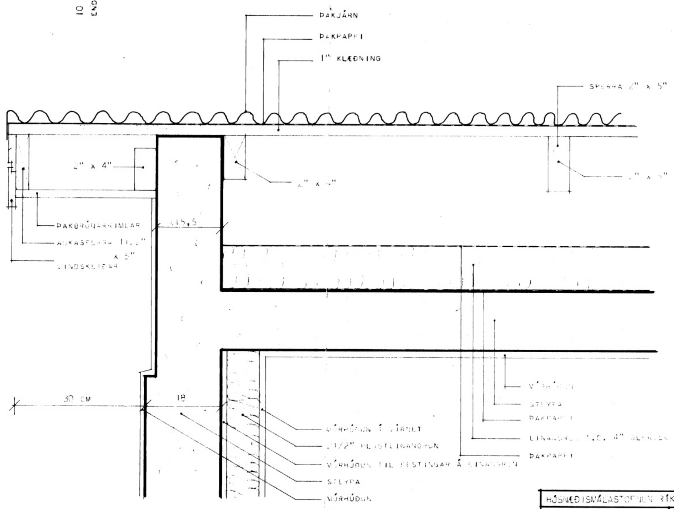
LÓDRÉTT SNEIDING Í PAKBRÓN VÍÐ GAFL.
