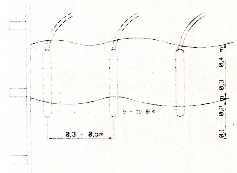
SKÝRINGAMYND: TITRUN STEYPU Í VEGGI
