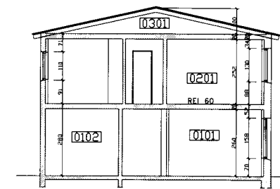
SNID A-A M=1:100
