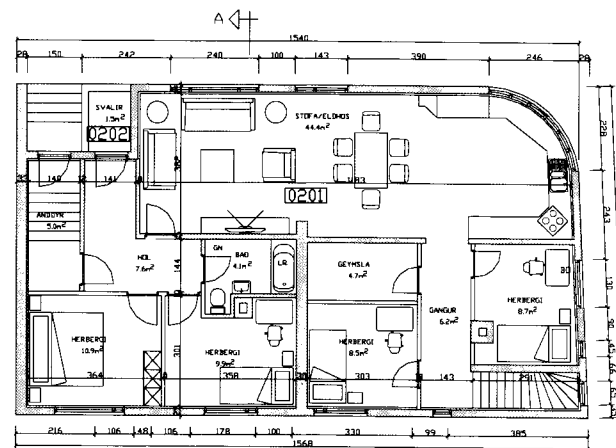
GRUNNMYND 2. HÆÐ M=1:100
