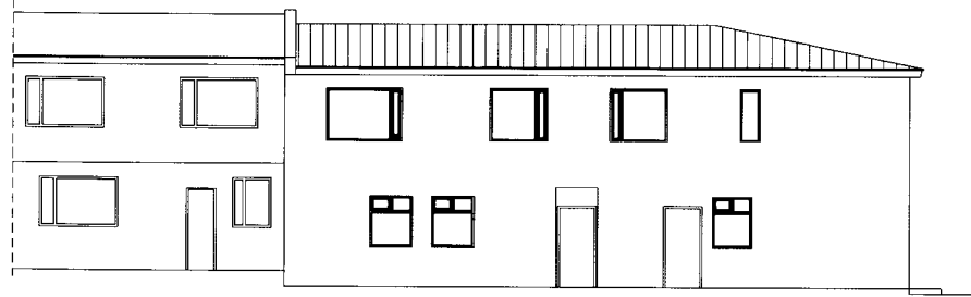
AUSTURHLID M=1:100
