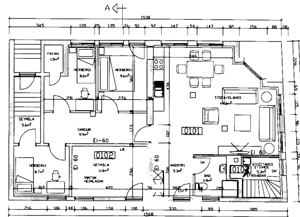
GRUNNMYND 1. HÆÐ M=1:100
