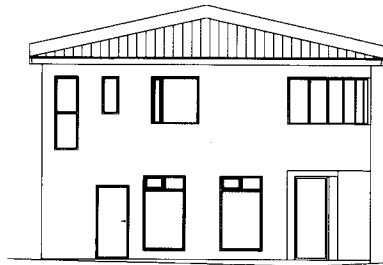
NORÐURHLID M=1:100
