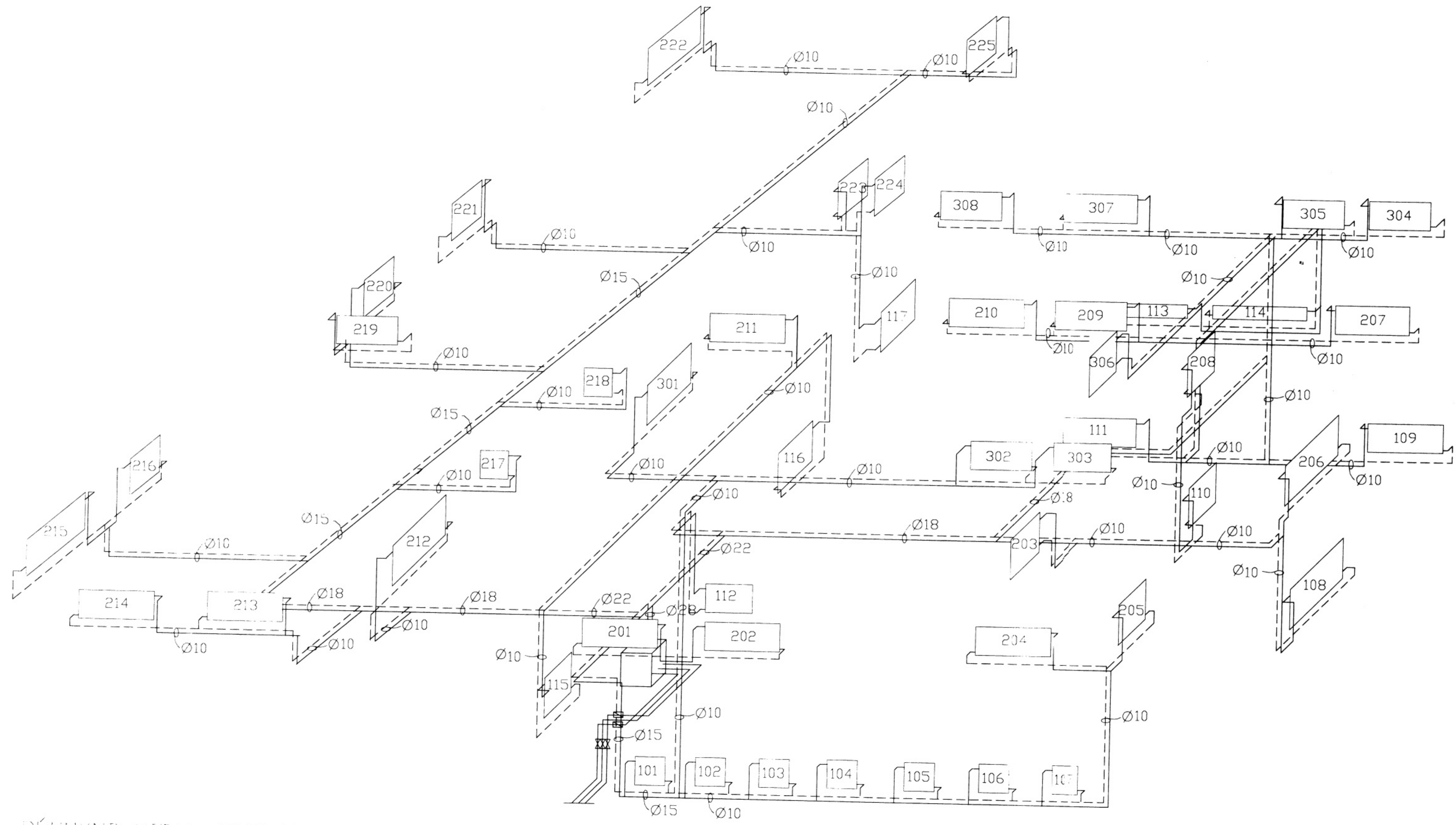
RÚNNYND HITALAGNIR M=1:50
